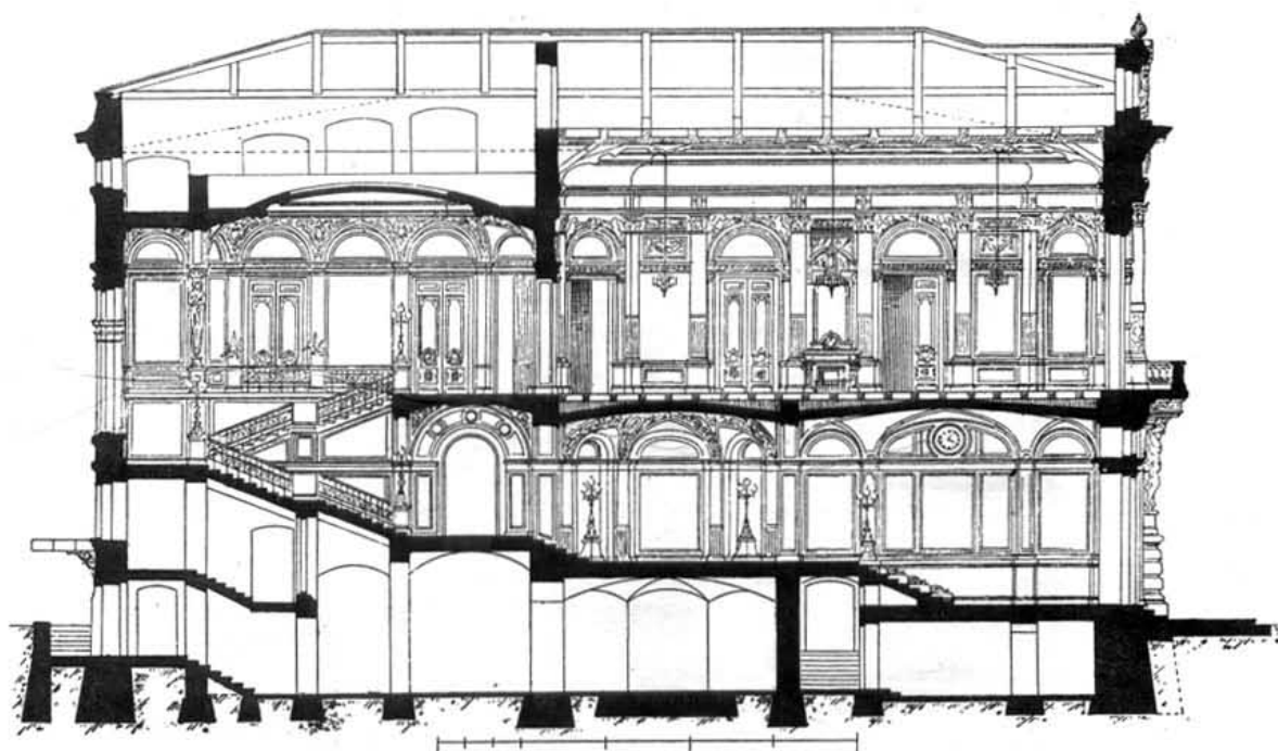
Продольный разрезъ.
