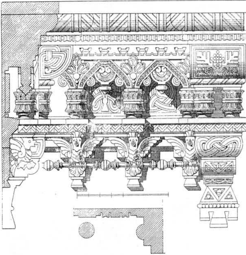
Деревянный карниз.
