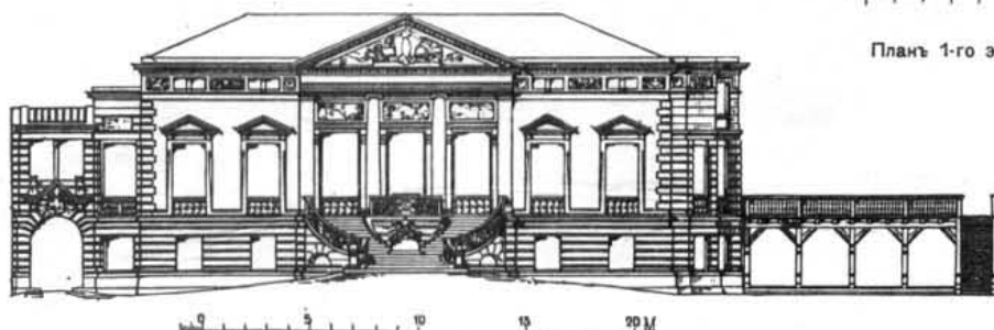
Фасадъ.
