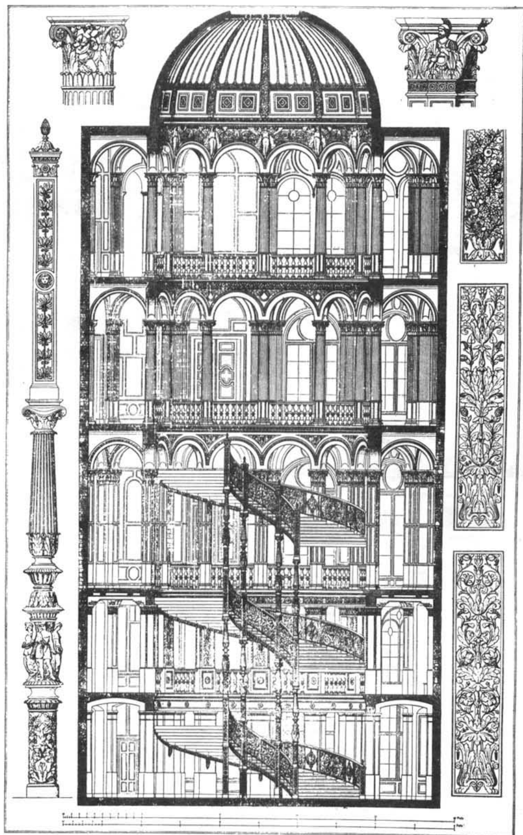
Разрѣзь и детали обработки мраморной лѣстницы.
