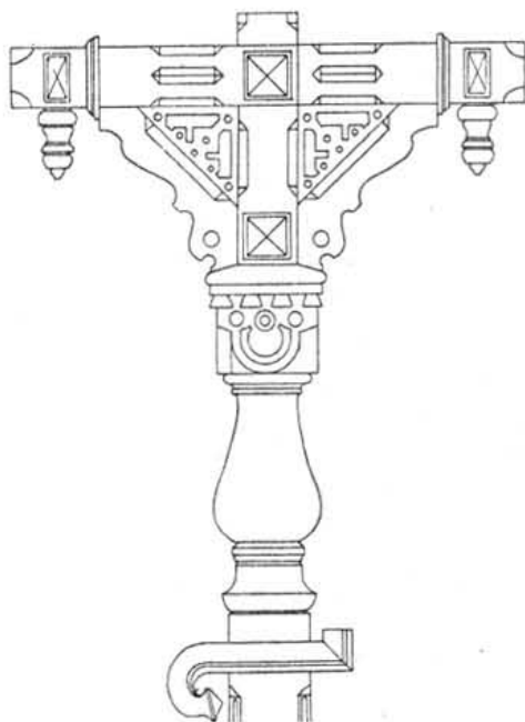
Столбъ навѣса.
