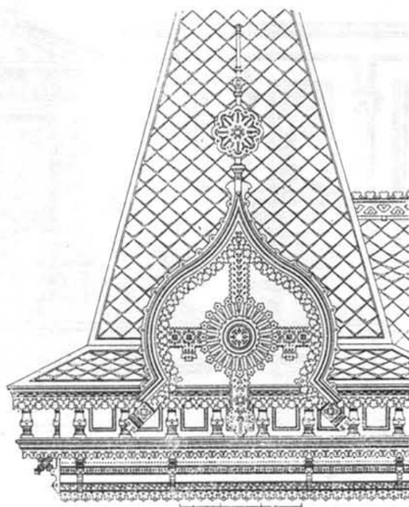
Фронтонъ башни. Проф. Арх. А. Н. Померанцевъ.
