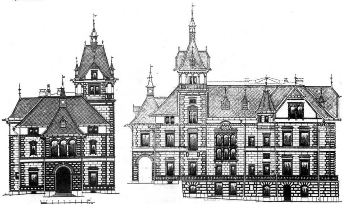
Фасады.
