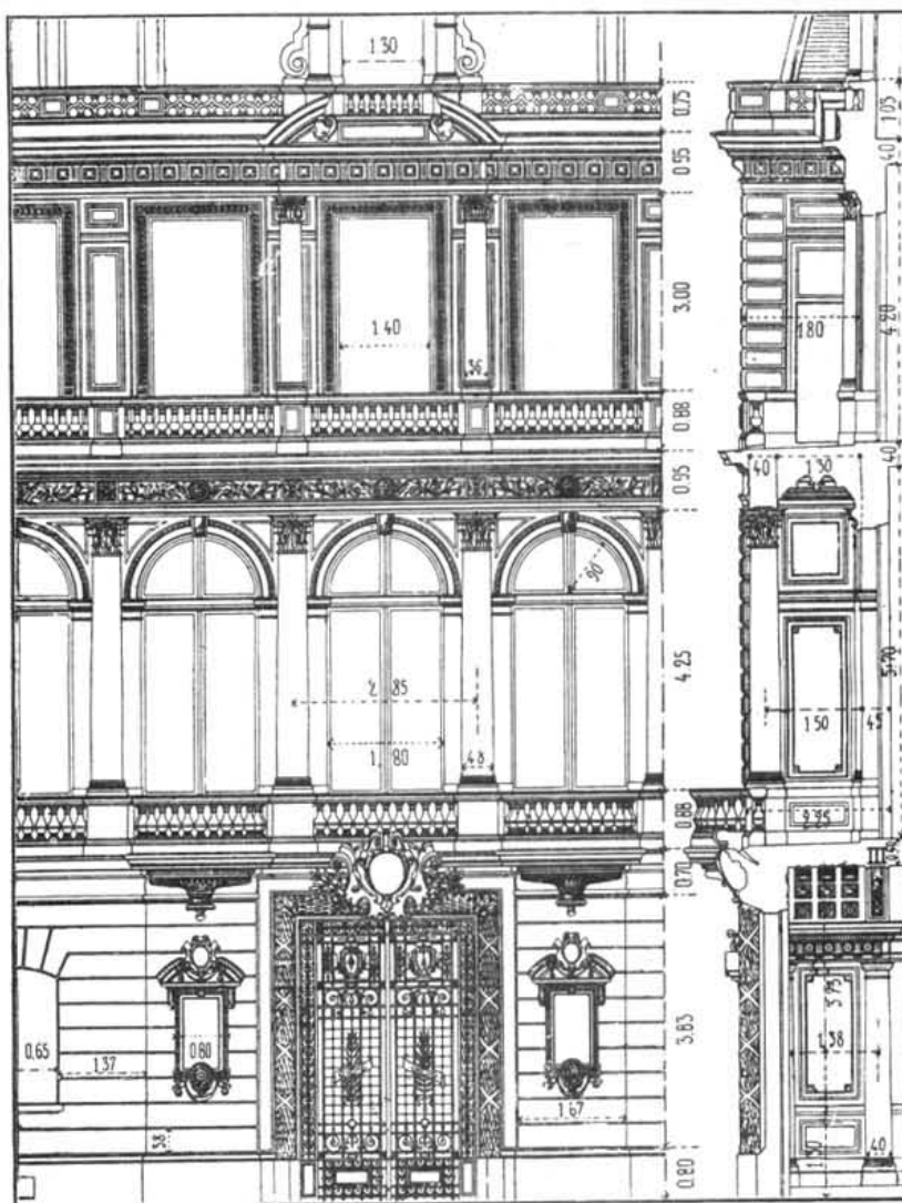
Деталь фасада.
