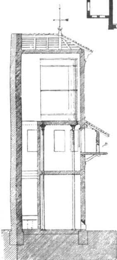
Разрѣзъ.
