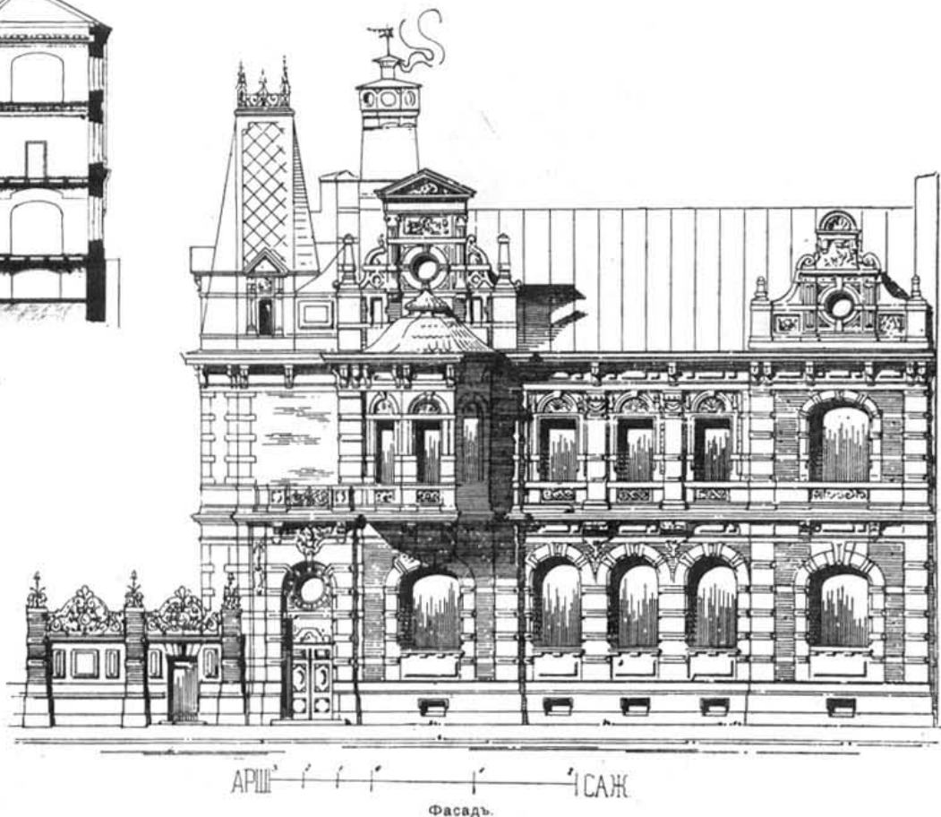
Фасадъ.
