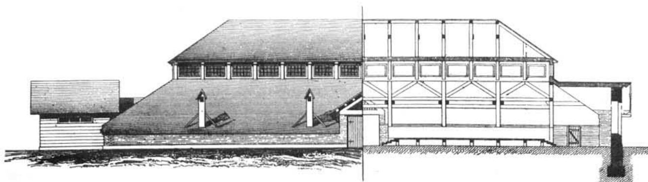
Продольный разрезъ.
