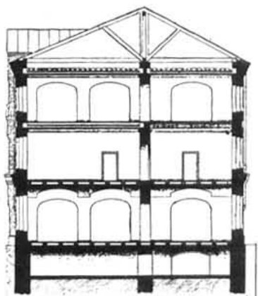
Разрѣзъ.
