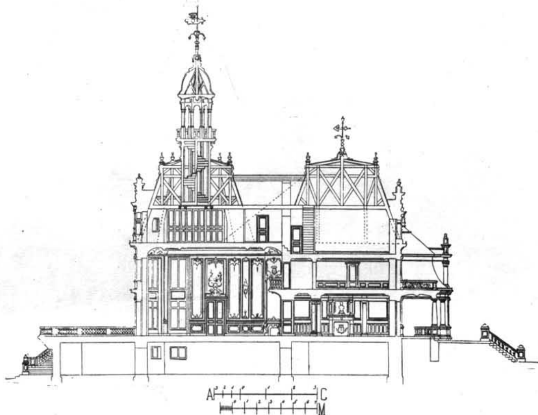
Поперечный разрез по главной оси.
