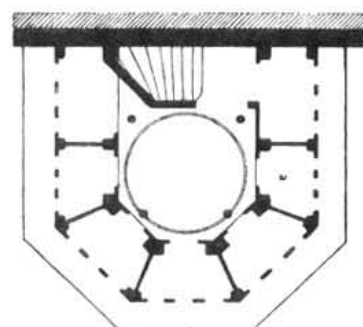
Планъ голубятни.
