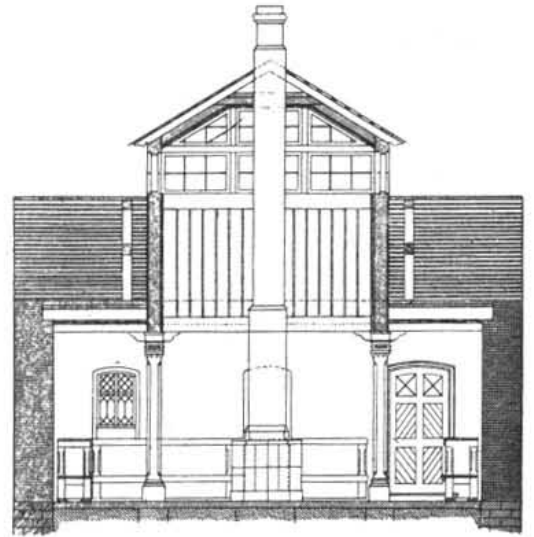
Продольный разрезъ молочной.
