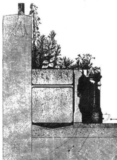
Детальный разръзъ парапета.
