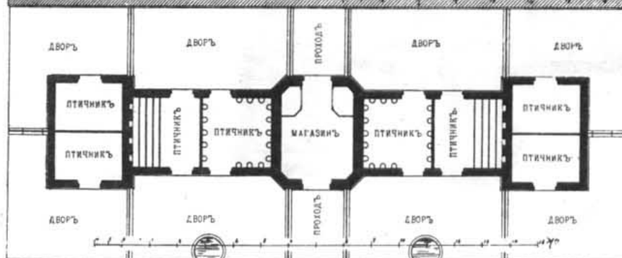
Детальный планъ.
