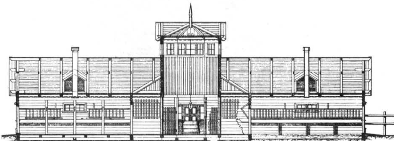
Продольный разрезъ конюшни.
