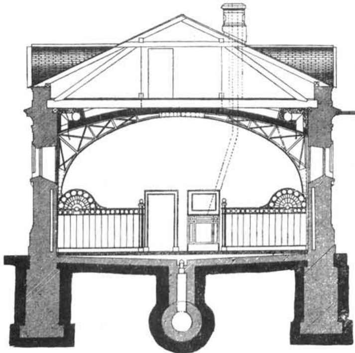
Поперечный разрезъ.
