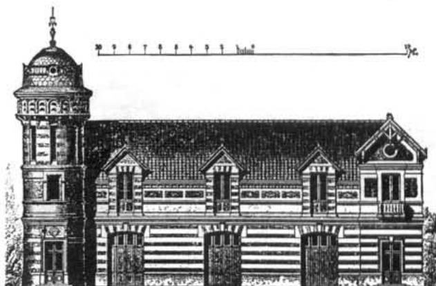
Главный фасадъ.
