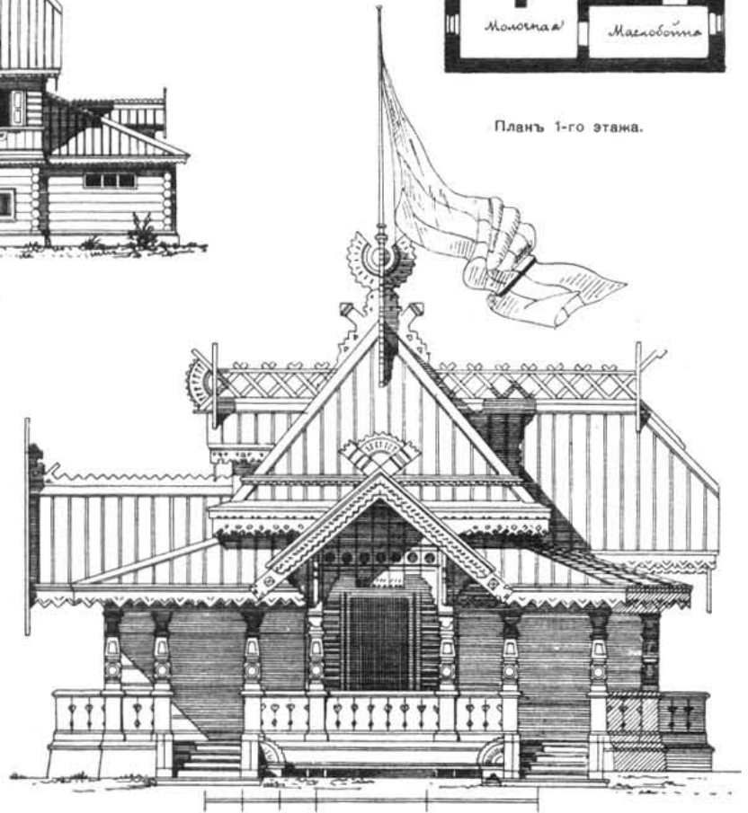
Главный фасадъ
