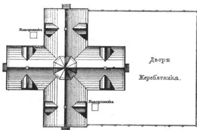
Генеральный планъ конюшни.
