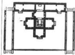
Планъ.
