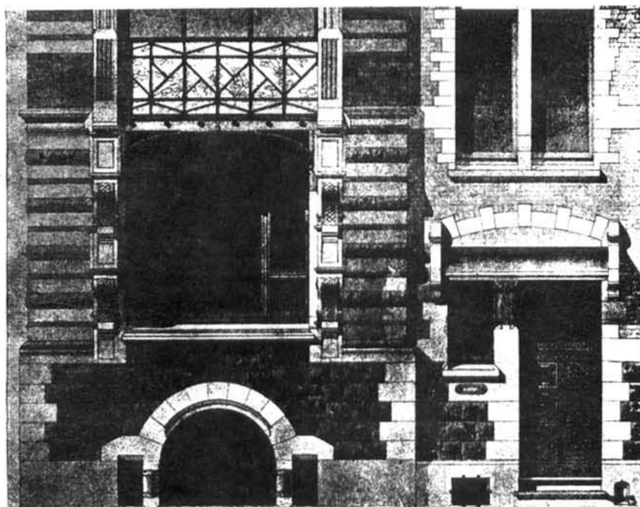
Разрѣзъ и деталь фасада.
