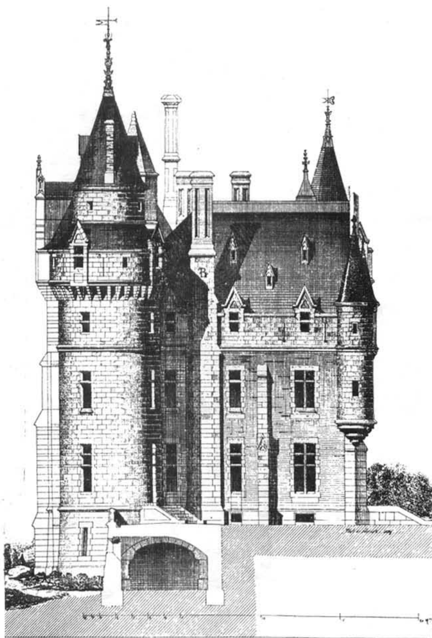
Левый боковой фасадъ.
