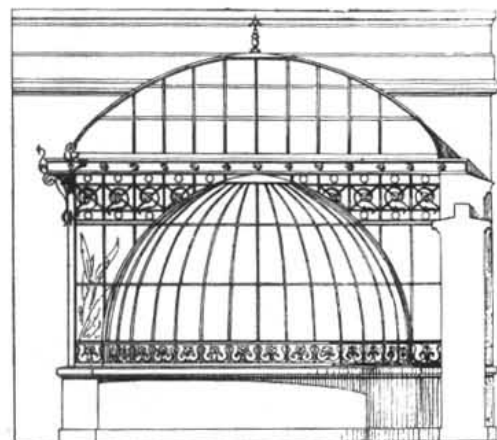
Поперечный разръзъ.
