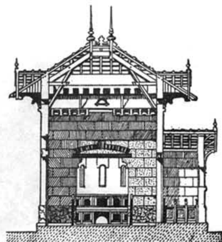
Поперечный разрътъ.
