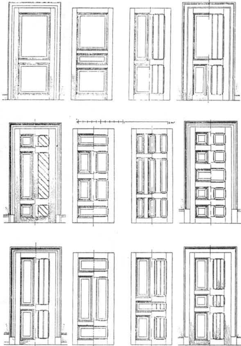
Одно—двустворные двери по Krauth'y.
