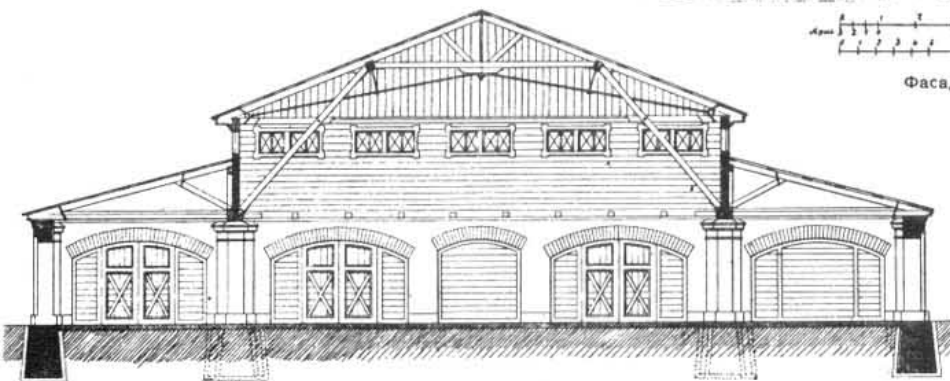
Поперечный разръзъ.
