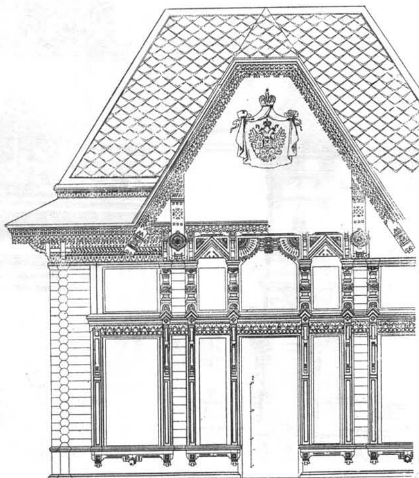
Фронтонъ окна.
