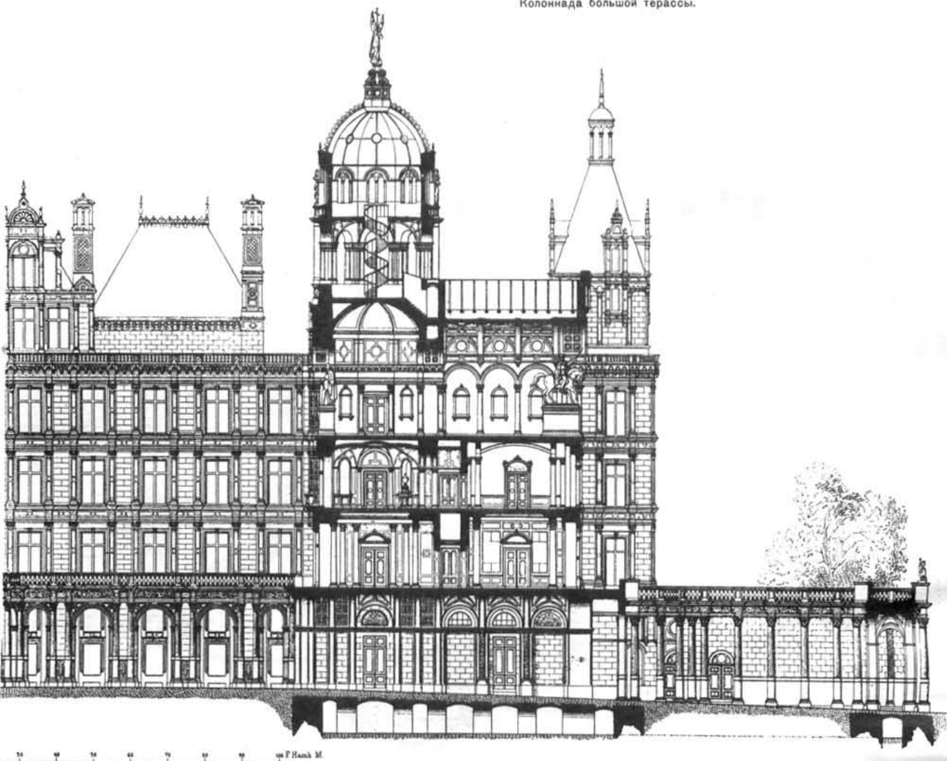
Разрѣзъ и юго-восточный фасадъ двора.
