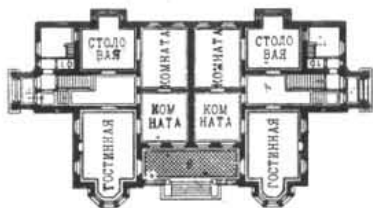
Планъ.
