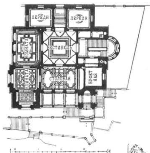
Планъ 1-го этажа.
