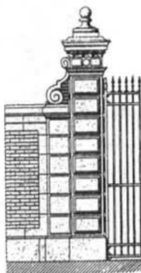
Столбы оградъ. Виллы въ Neuilly, бл. Парижа.
