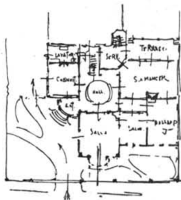
Планъ.
