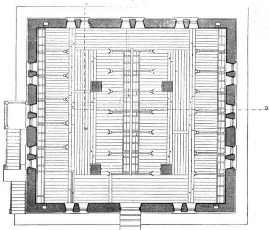
Планъ коровника.
