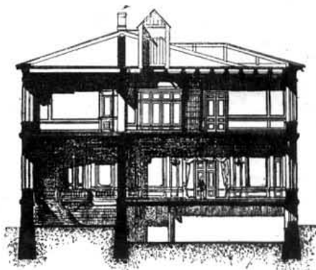
Разрѣзъ.
