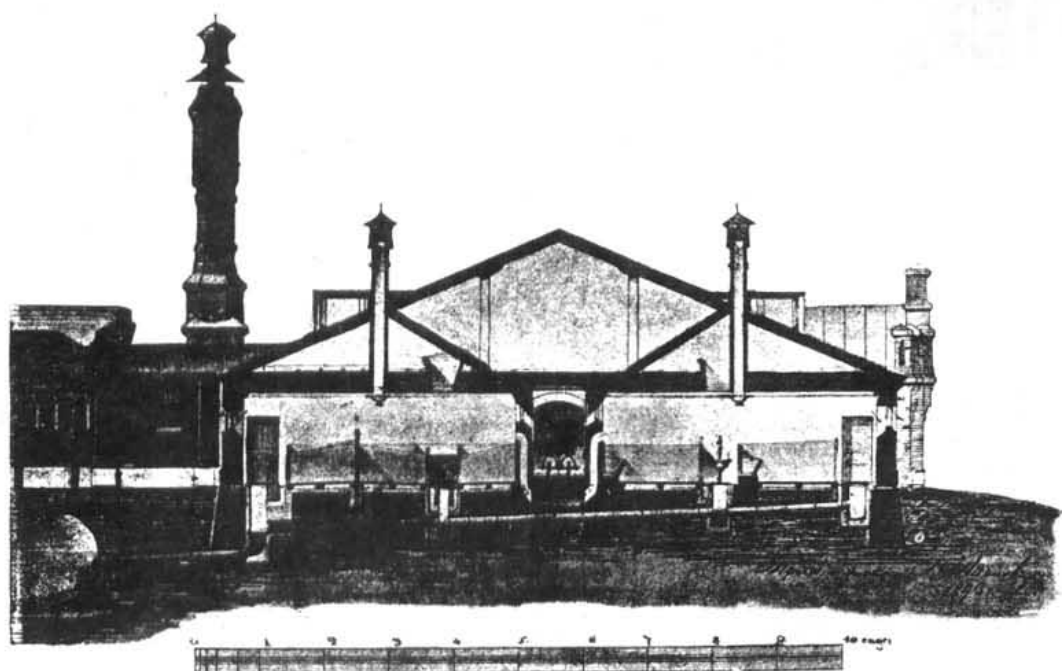
Разръзъ коровника.
