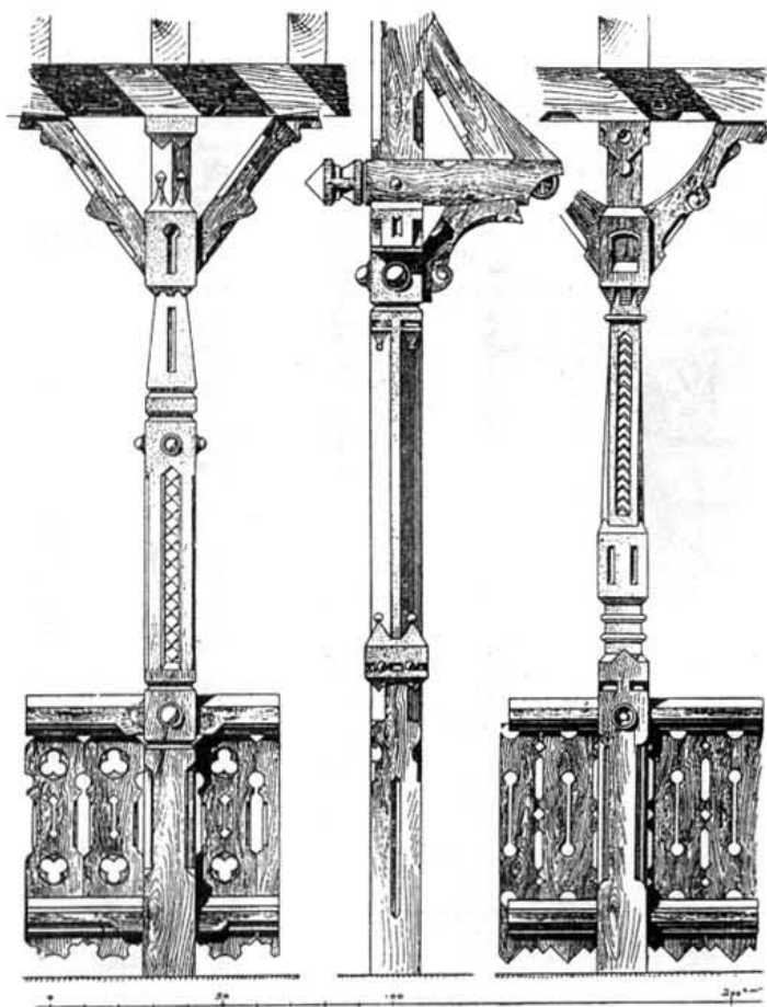
Дерев. столбы и колонны по Krauth'y и Meyer'y.
