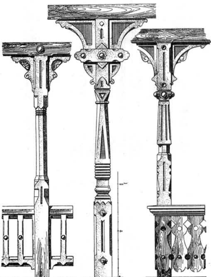
Дерев. столбы и колонны
