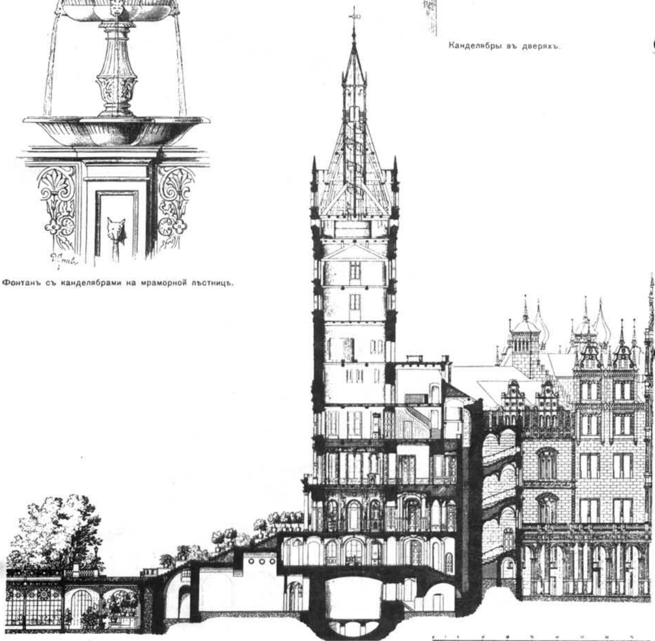
Разрѣзъ и сѣверо-восточный фасадъ.
