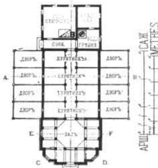
Планъ.
