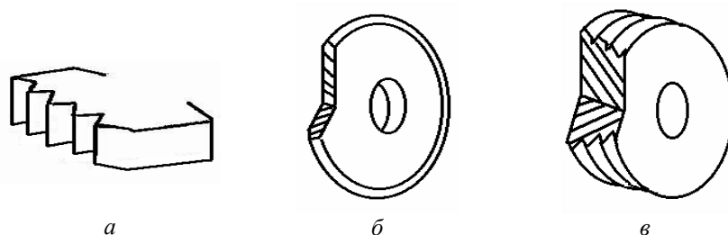
Рис. 5 Фасонные резцы: а – призматический многониточный; б – круглый (дисковый) однониточный; в – дисковый многониточный
