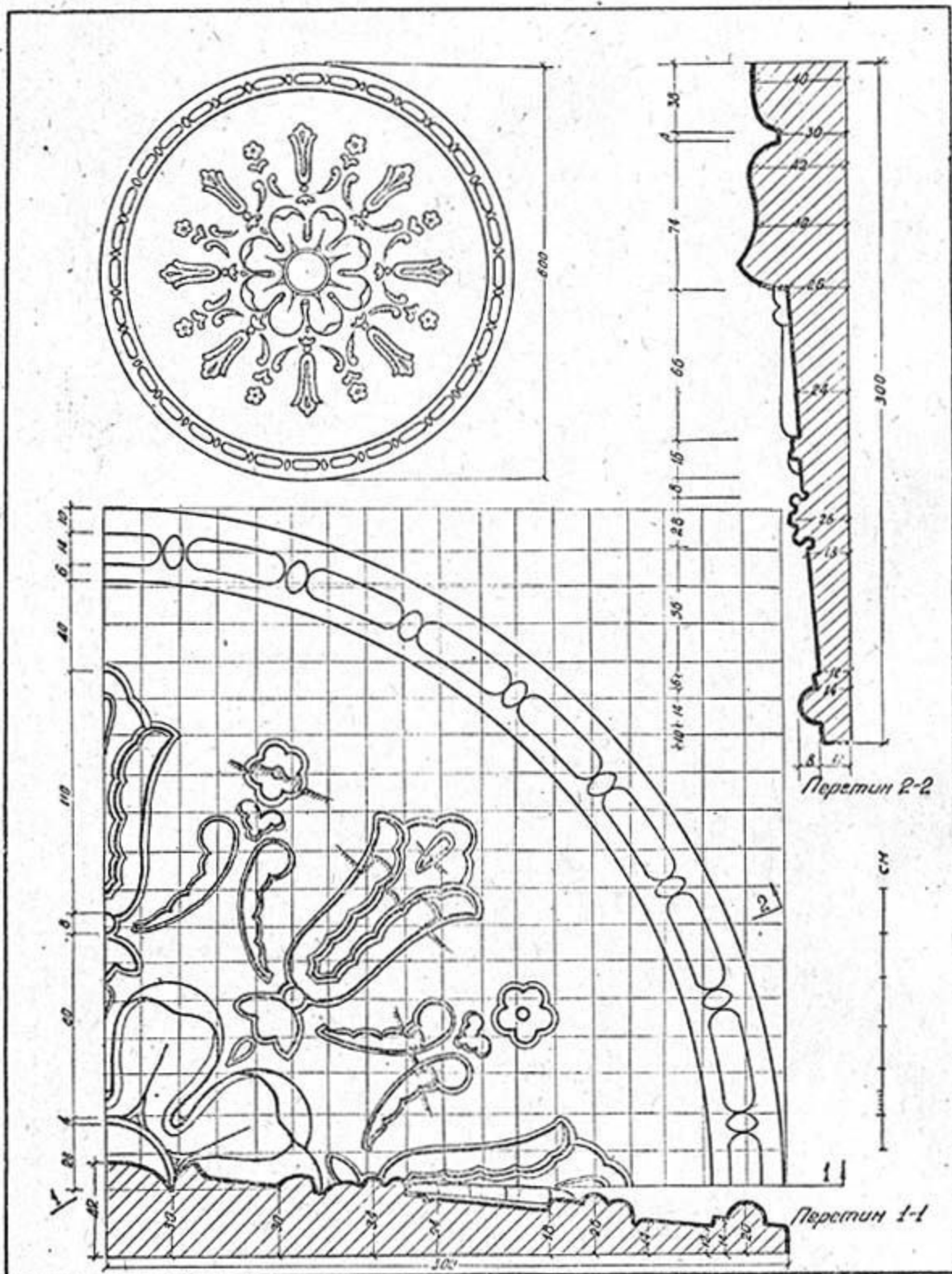
Розета для стелі ліпна.
