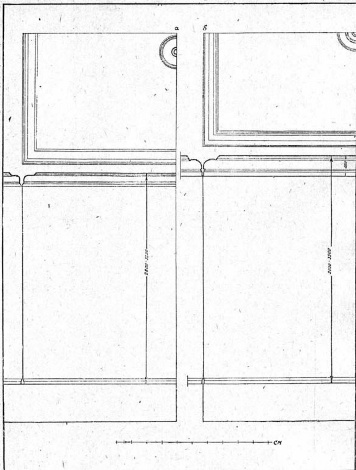
а—розвертка стін і стелі: 1—карниз (аркуш 2-б); 2—розвертка (аркуш 13). б—розвертка стін і стелі: 1—карниз (аркуш 2-а); 2—розета (аркуш 15).
