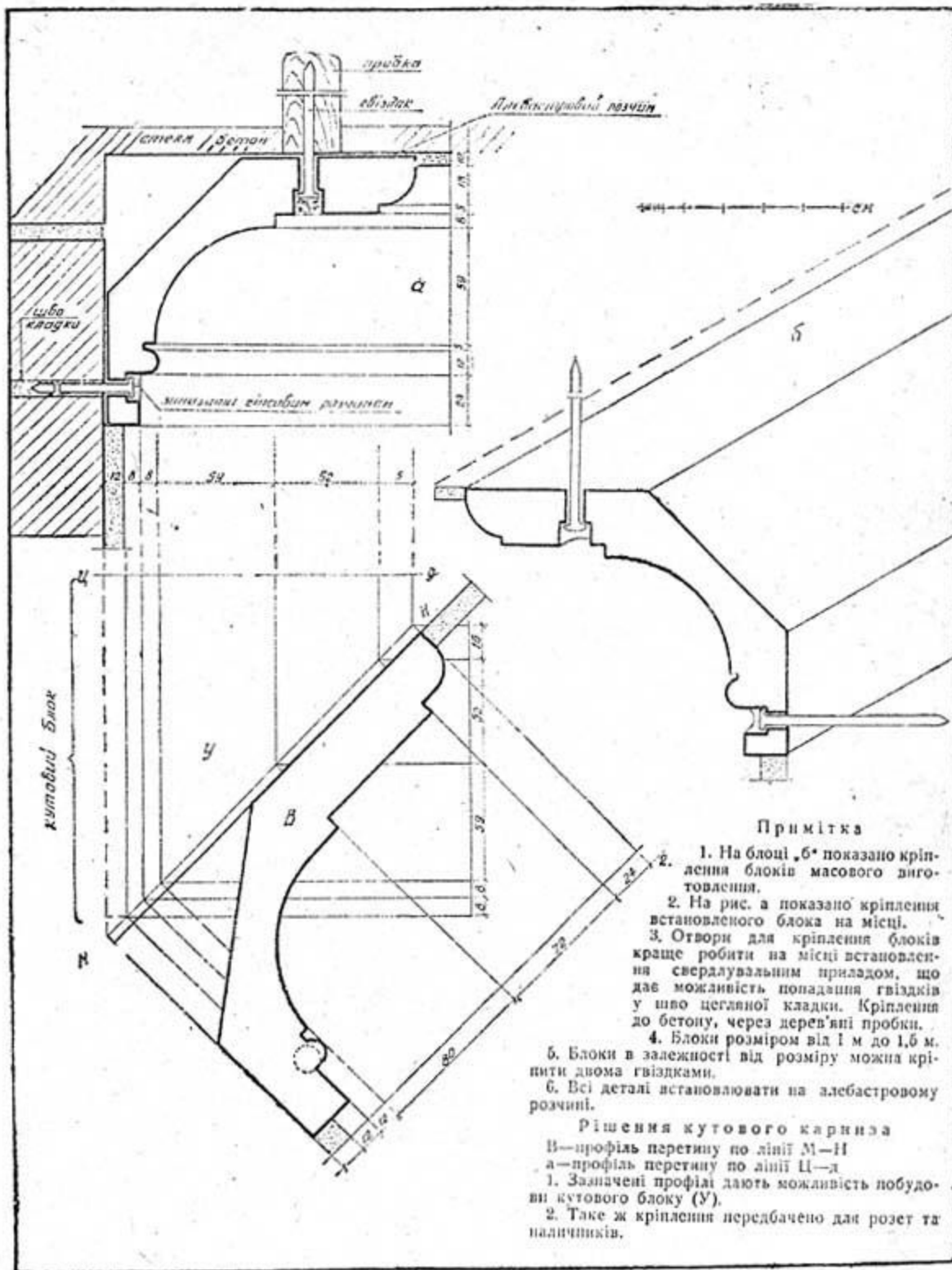
Приклад конструювання і кріплення блочних карнизів розет і наличників масового виготовлення.
