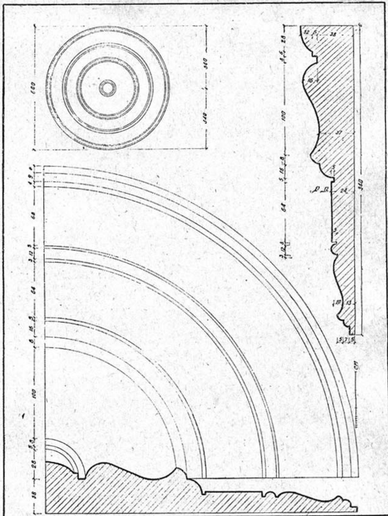
Розета тягнута для стелі.
