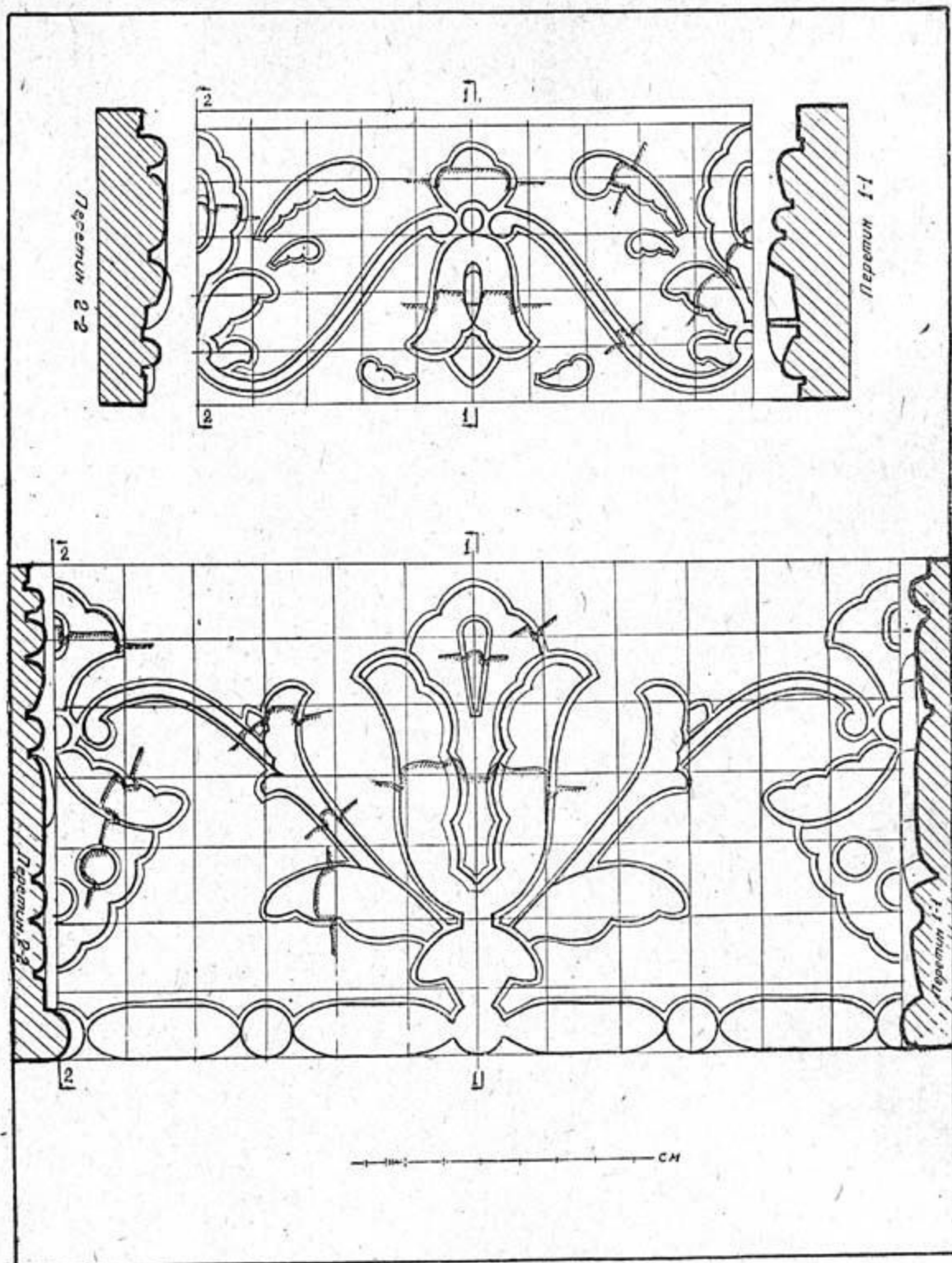
Блоки зіплення карнизів (аркуші 7 та 5-а).
