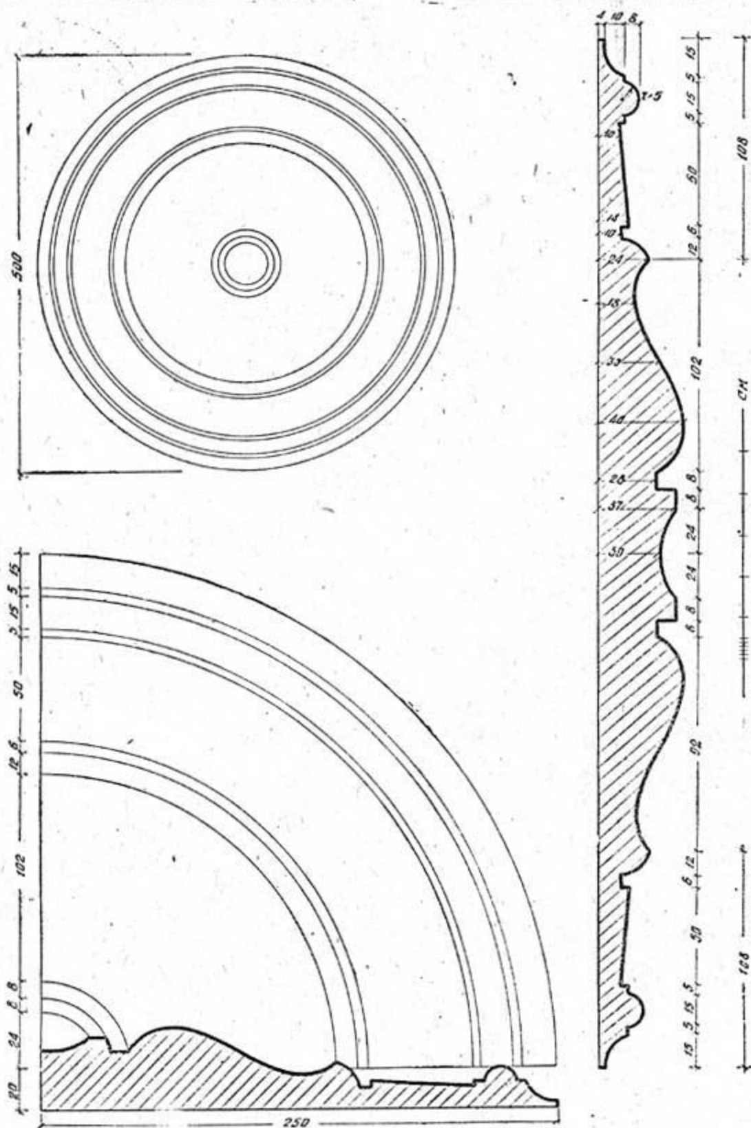
Розета тягнута для стелі.
