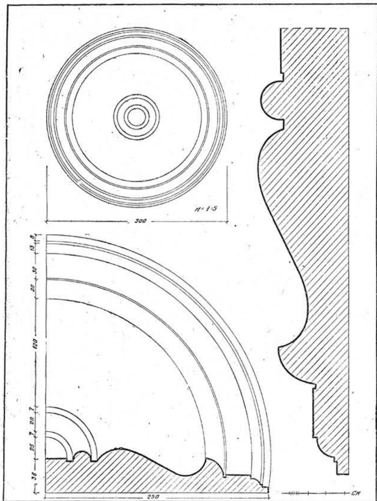
Розета тягнута для стіні.
