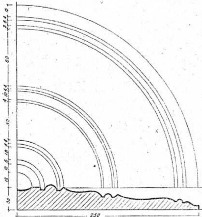
Розета тягнута для стелі.
