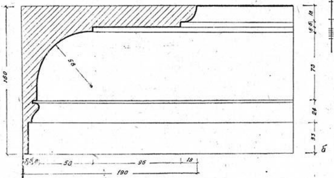
Карнизи тягнуті для житих приміщень.
