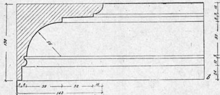
Карнизи тягнуті (мал).
