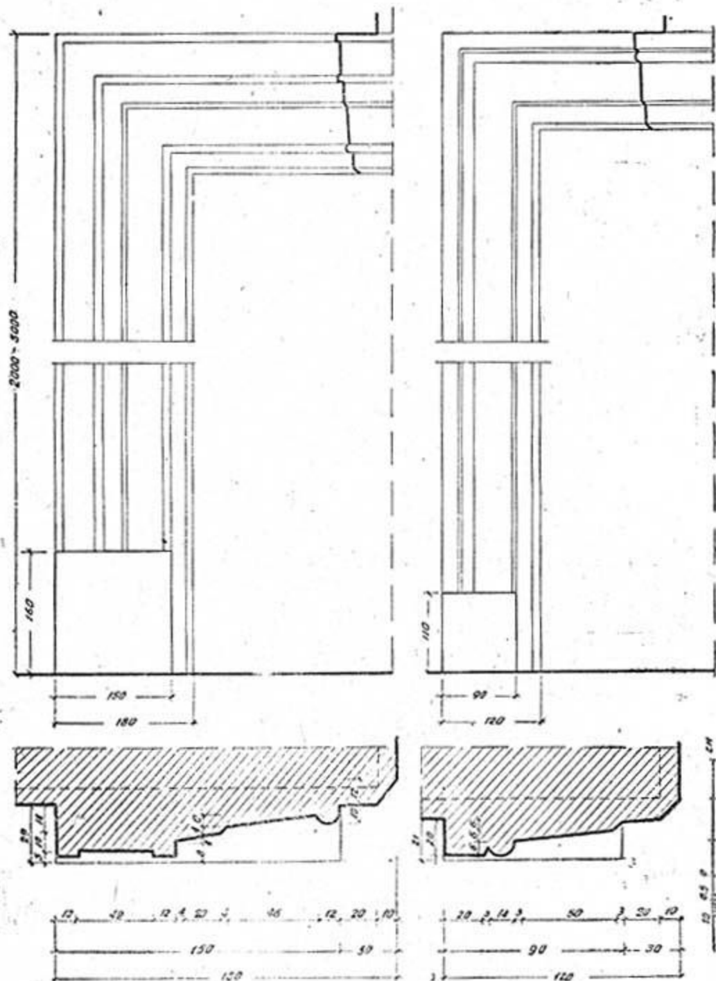
Наличники для дверей, тягнуті.
