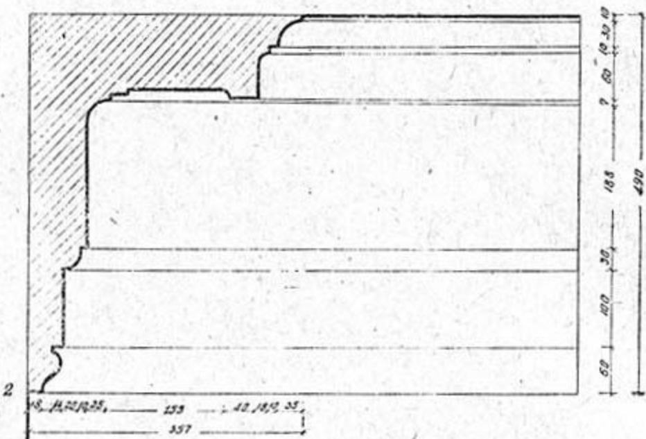
1—стена; 2—карниз; 3—розета (аркуш 13).
