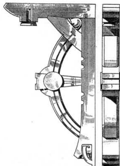
Мотивы деревянных консолей. По Dorschfeldt'y.
