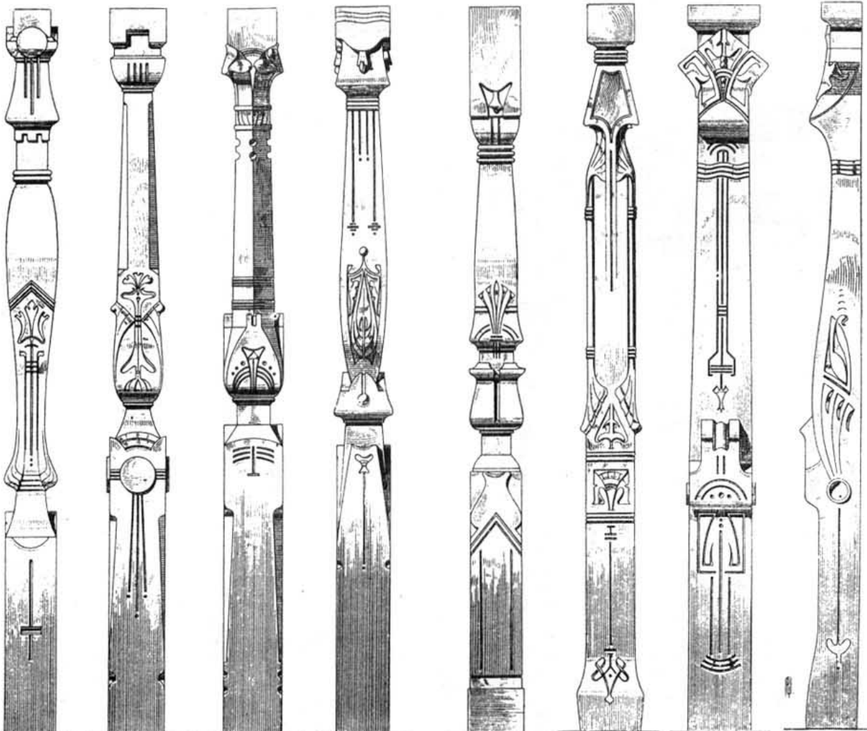
Дерев. колонны и столбы (по В. Dorschfeldt'y).
