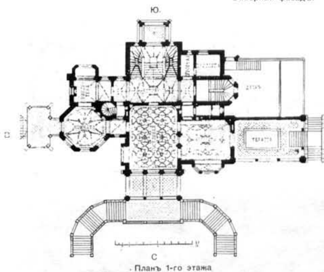
Планъ 1-го этажа
