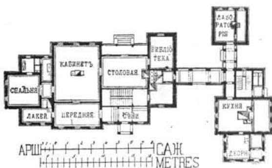
Планъ 1-го этажа.
