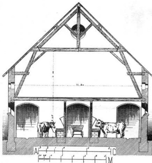
Поперечный разрезъ.
