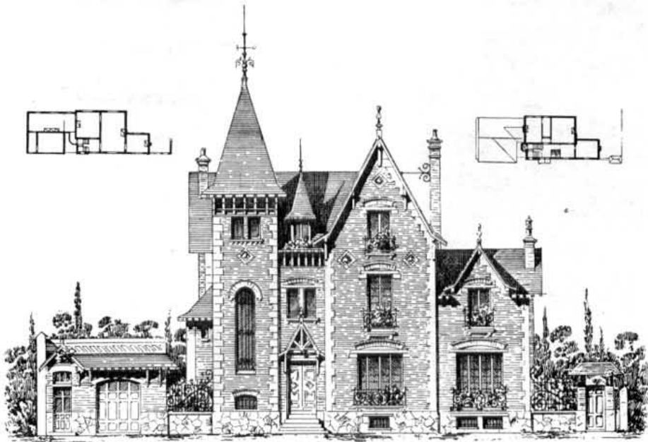
Фасадъ.
