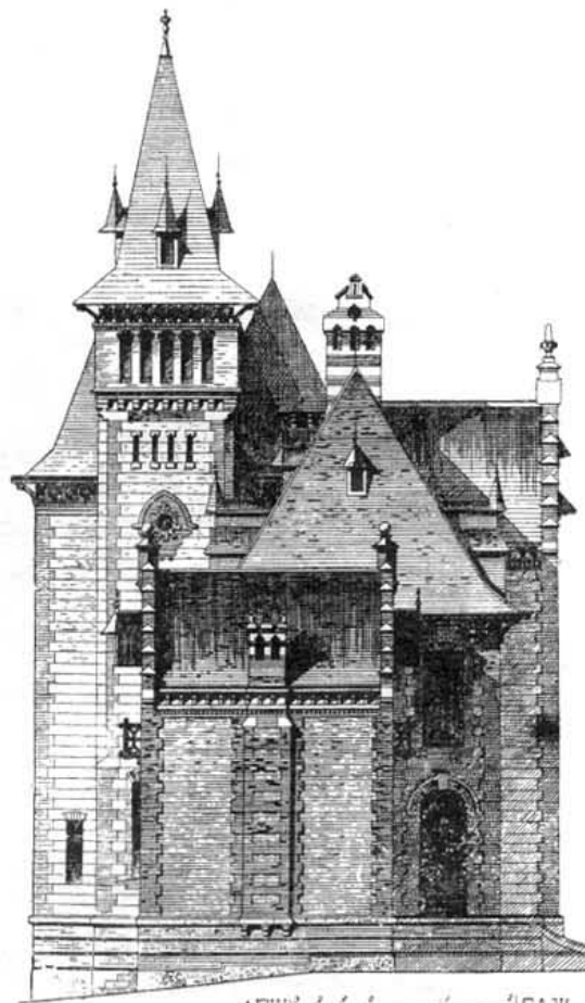
Боковой фасады.
