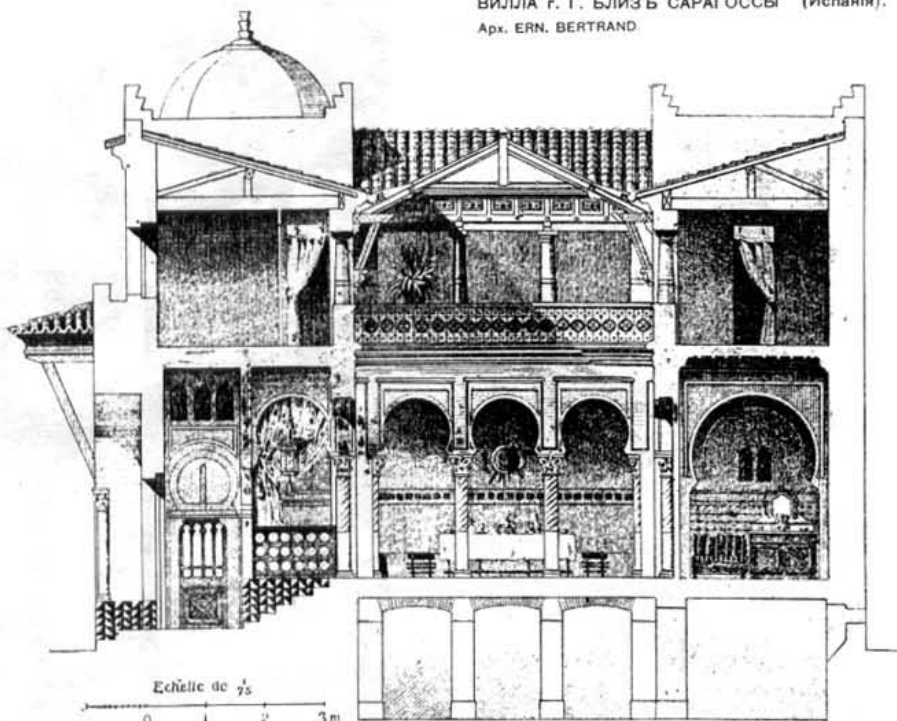
Разрѣзъ.
