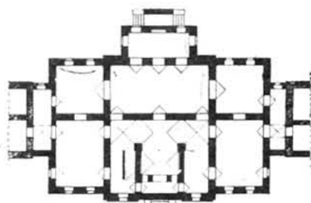
Планъ подвала.
