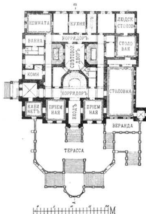
Планъ 2-го этажа.
