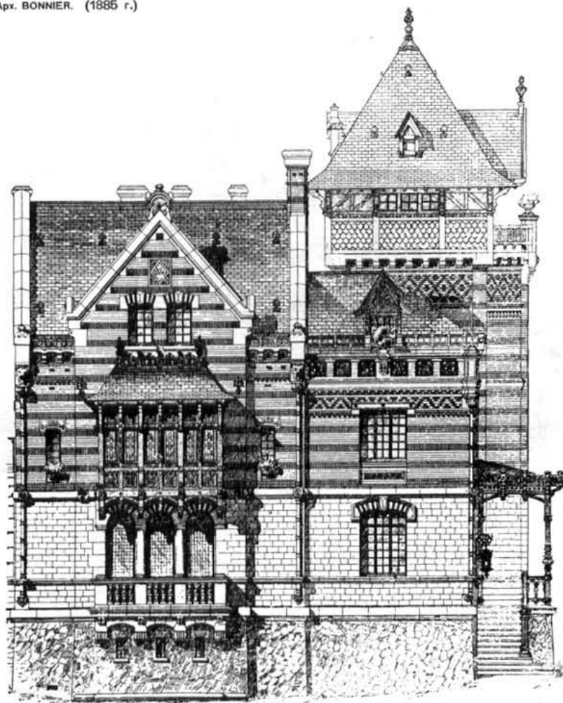
Боковой фасадъ.
