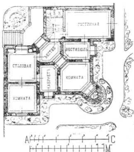
Планъ 1-го этажа.
