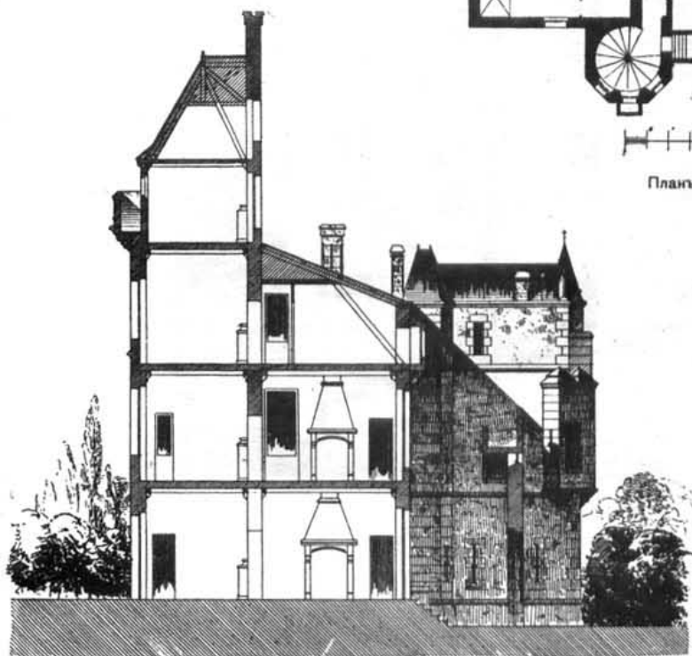
Разрѣзъ.
