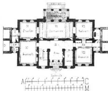
Планъ 1-го этажа.
