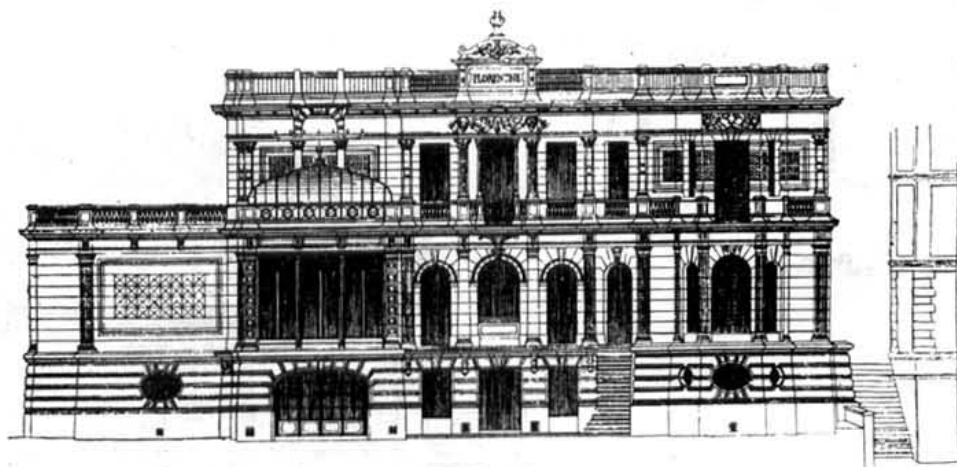
Южный фасадъ
