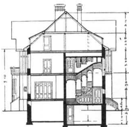
Разрѣзъ.
