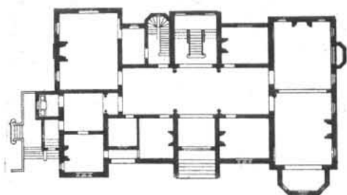
Планъ 1-го этажа.
