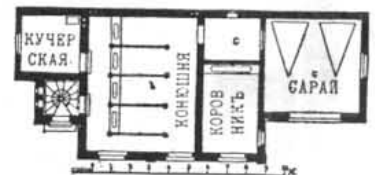
Планъ.
