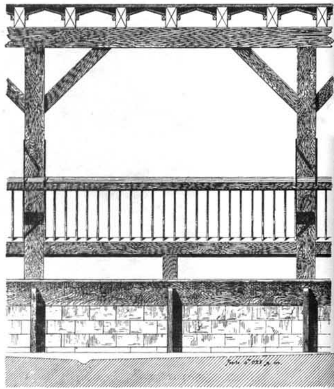
Детали устройства кормовыхъ ящичковъ.
