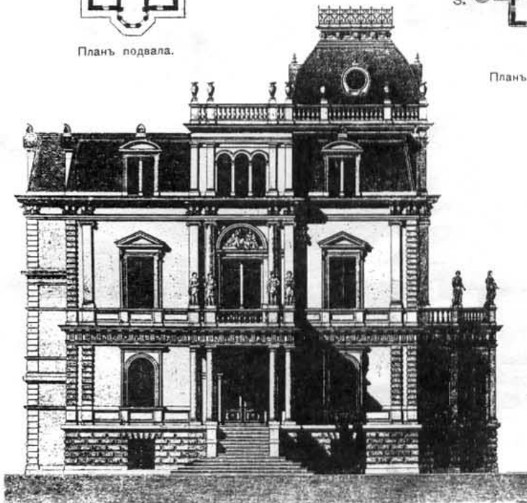
Западный фасадъ.
