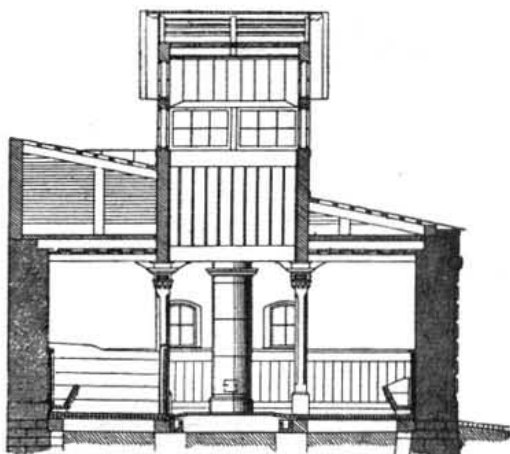
Поперечный разрезъ телятника.
