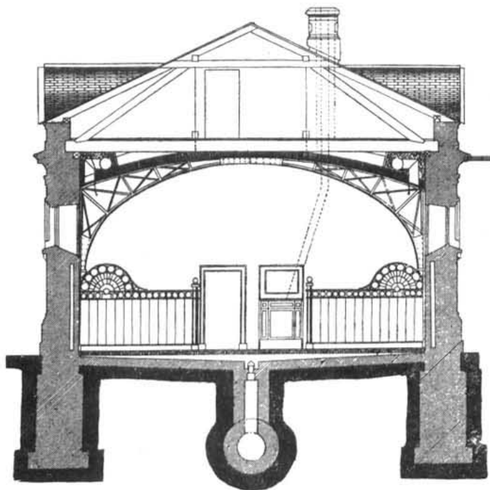
Поперечный разрезъ.
