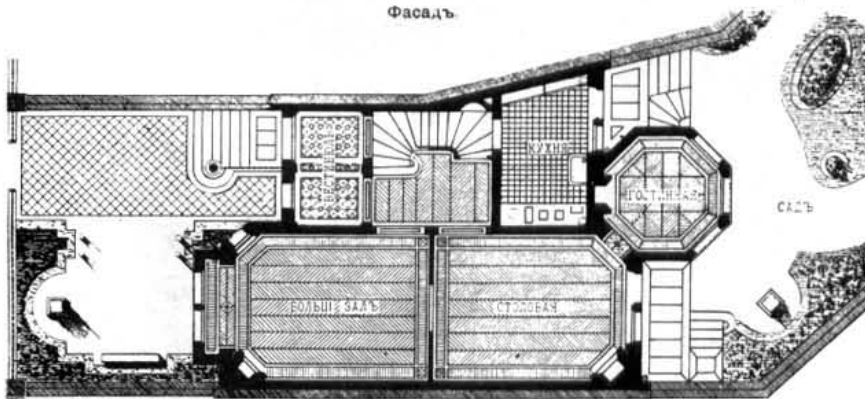
Планъ I-го этажа.
