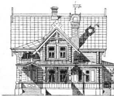
Боковой фасадъ.
