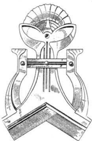
Деревянные акротеры. Арх. R. Dorschfeldt.
