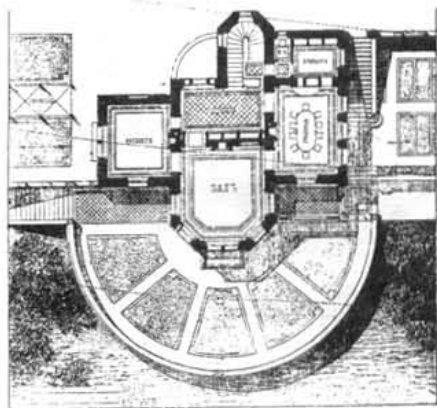
Планъ.
