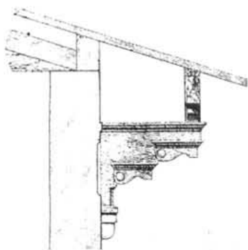
Деталь карниза на консолях.
