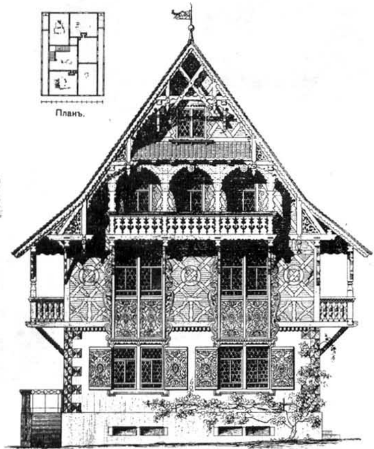
АРШ. 1 САЗ. 1 МЕТРЕС. Фасадъ.
