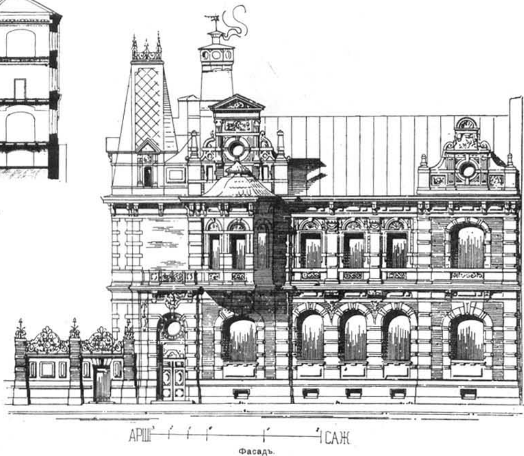
Фасадъ.
