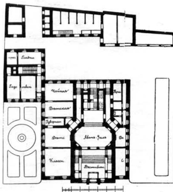
Планъ 1-го этажа.
