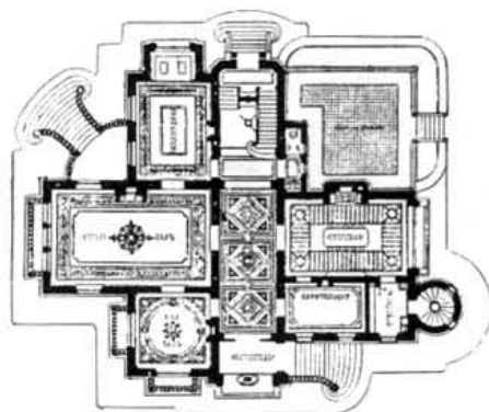
Планъ полуподвала.
