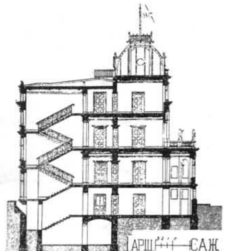
Разрѣзь по линіи С. Ю.
