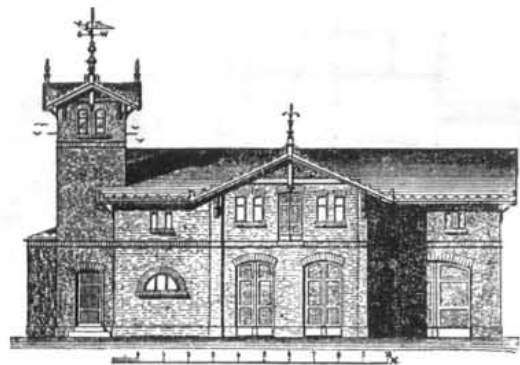
Фасадъ.
