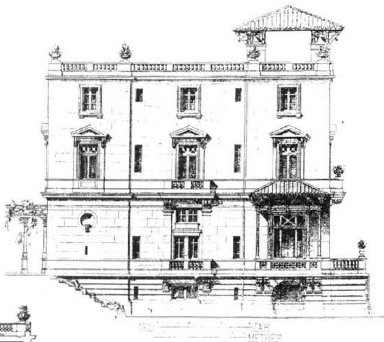
Боковой фасад (западный).
