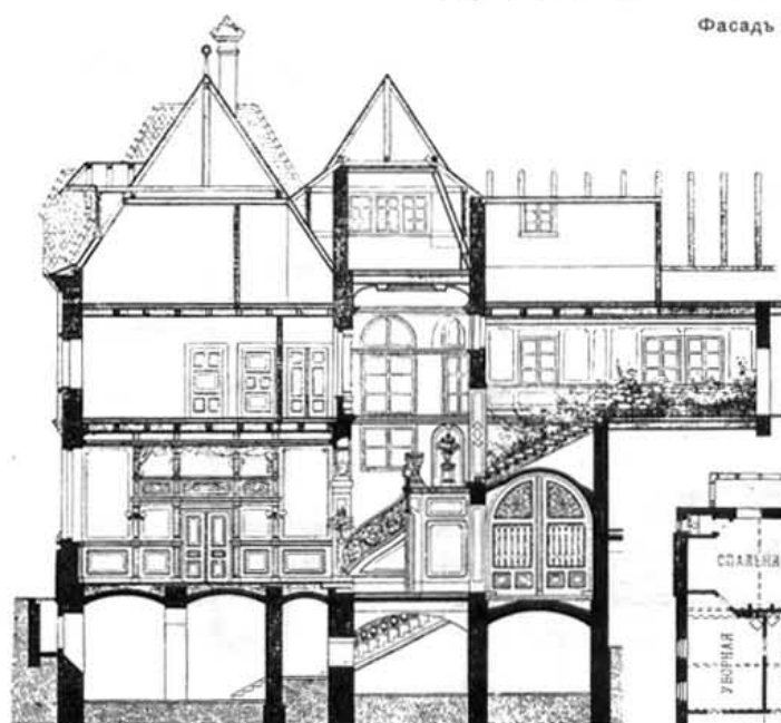
Разрѣзъ.
