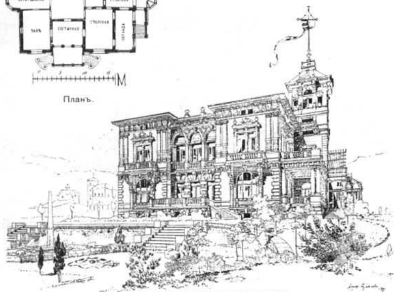
Перспективный видъ.
