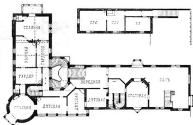
Планъ 2-го этажа.
