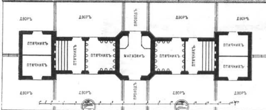
Детальный планъ.
