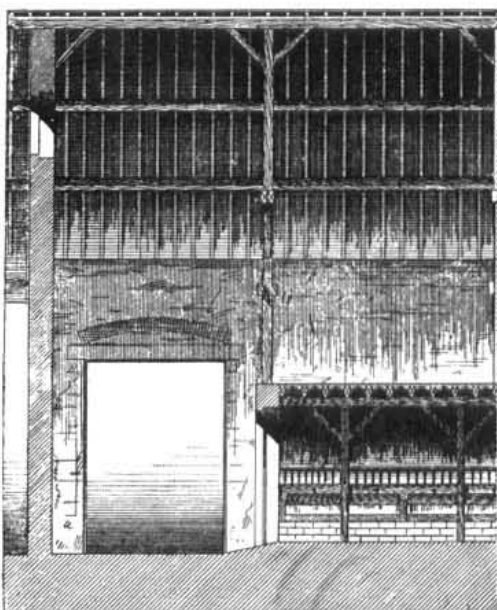
Часть продольного разреза.
