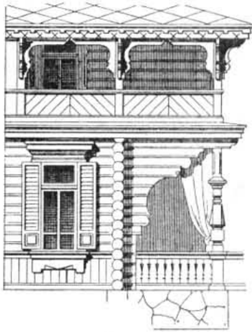
Деталь.
