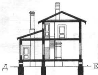
Разрѣзъ.
