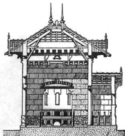
Поперечный разрътъ.
