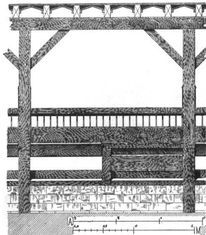
Главный фасадъ.
