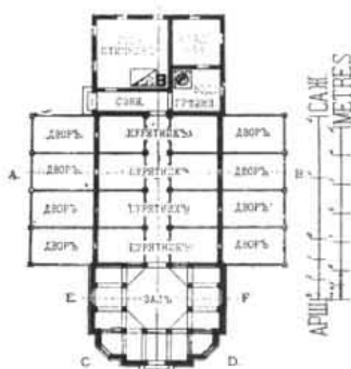
Планъ.
