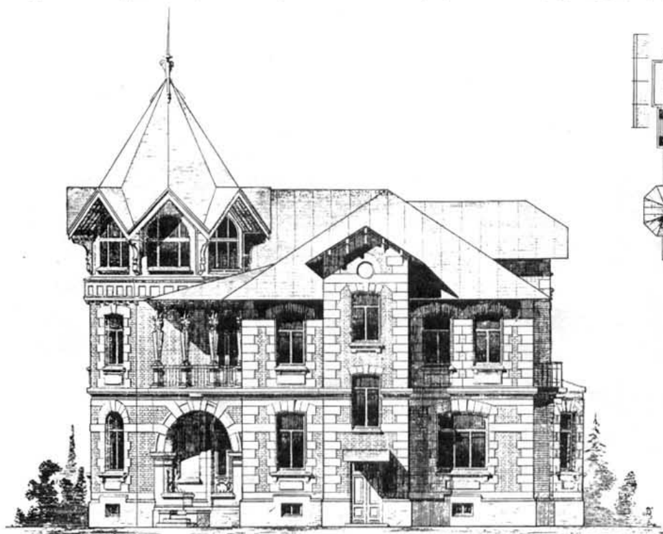
Западный фасадъ.
