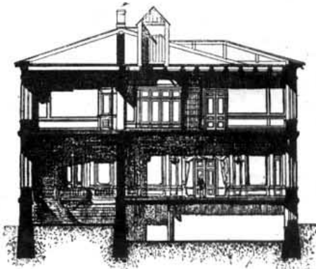
Разръзъ.
