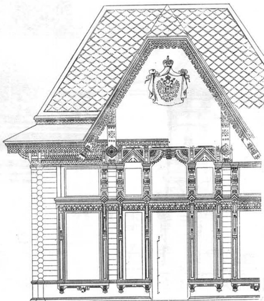
Фронтонъ окна.
