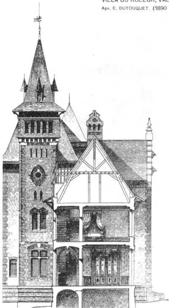
Поперечный разрезъ.
