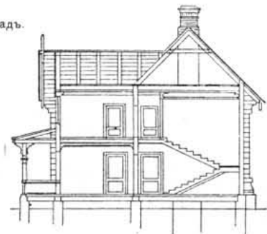
Разрѣзъ.
