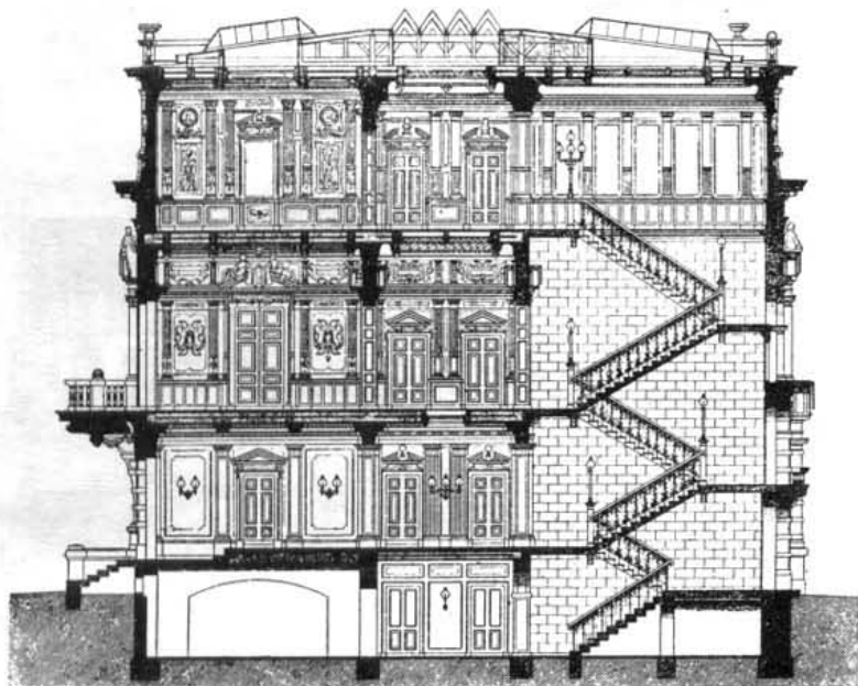
Разрѣзъ.
