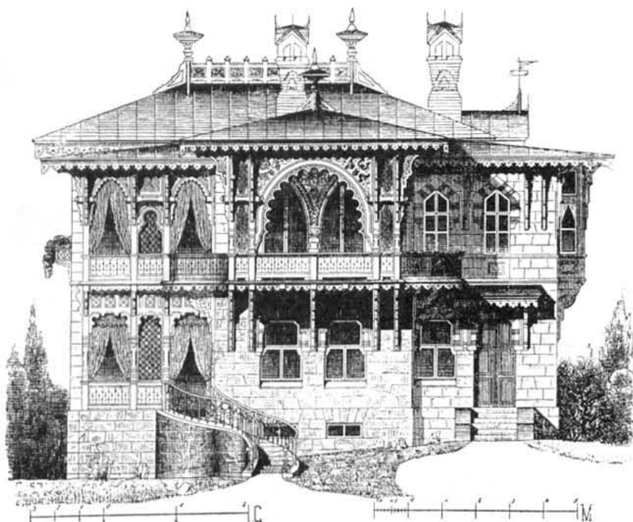
Фасадъ.
