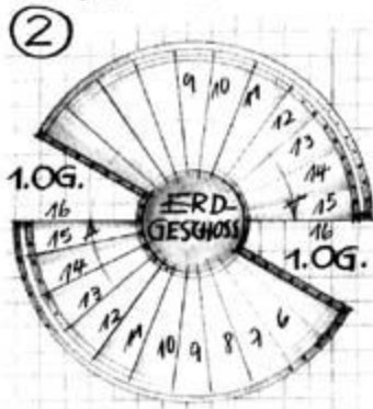
VOGELPERSPEKTIVE
