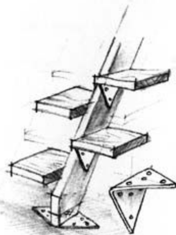
TRAGHOLM AUS STAHLROHR, STAHLBLECHWINKEL; HOLZSTUFEN,
