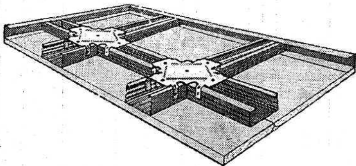
Рис. 7. Одноуровневый подвес потолка
