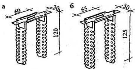
Рис. 8. Подвес прямой:
