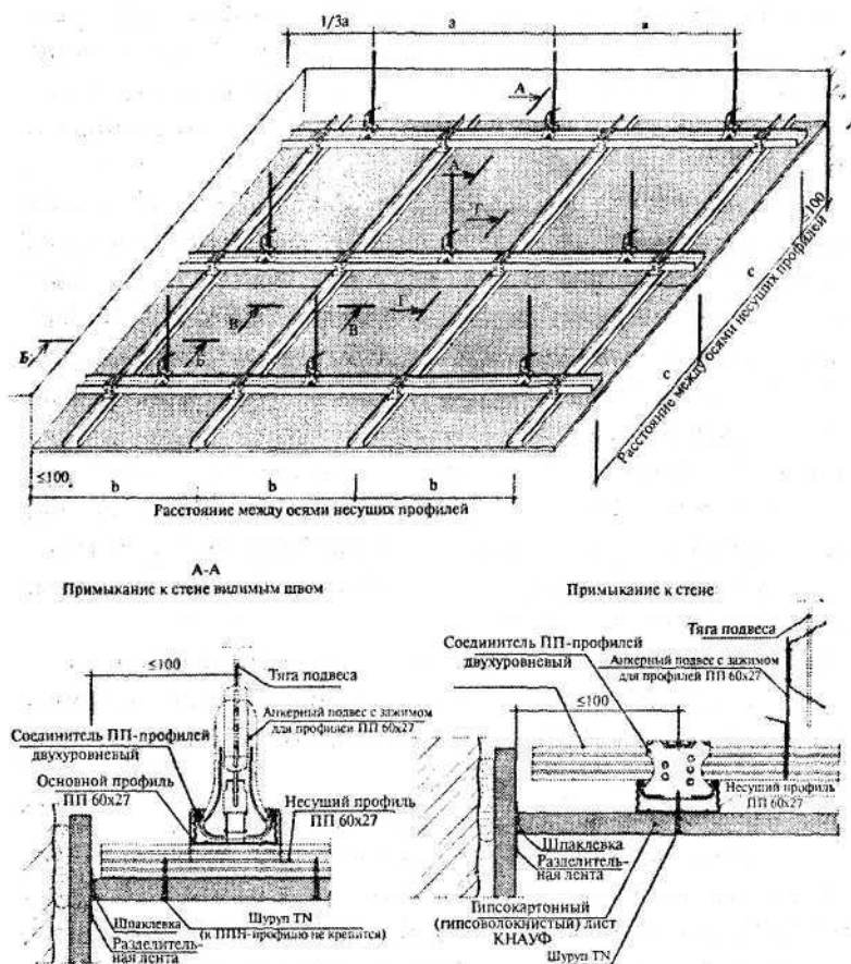
Рис. 5. Конструкция двухуровневого подвесного потолка Л112, (П212)
