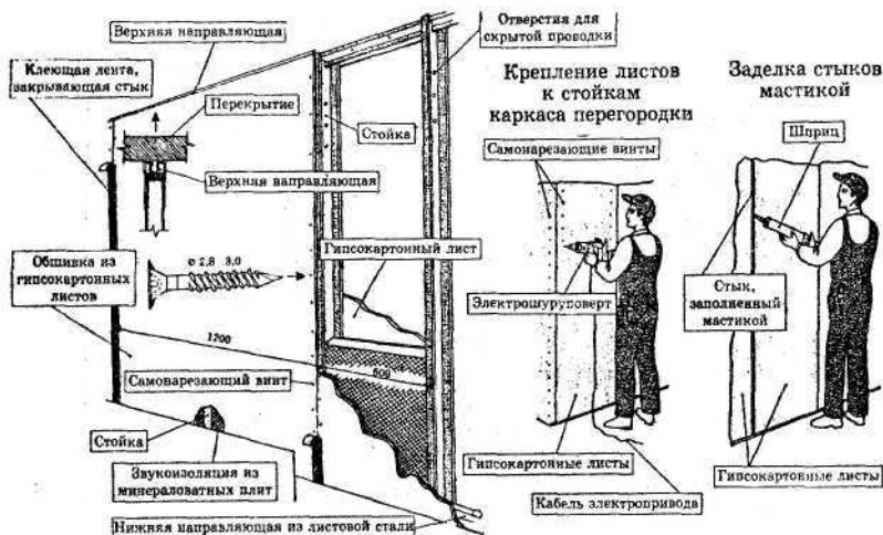
Рис. 3. Конструкция перегородки
