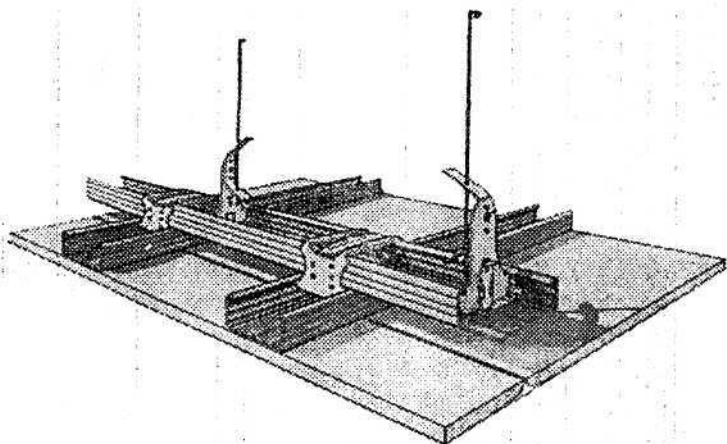
Рис. 6. Двухуровневый подвес потолка
