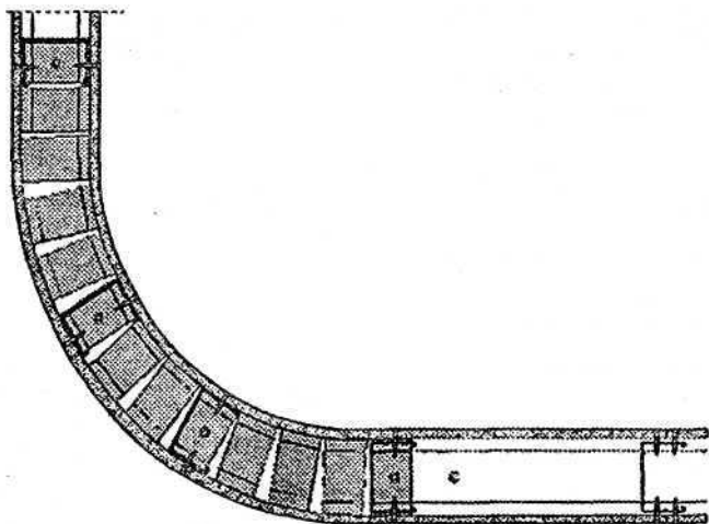
Рис. 12. Устройство криволинейной перегородки
