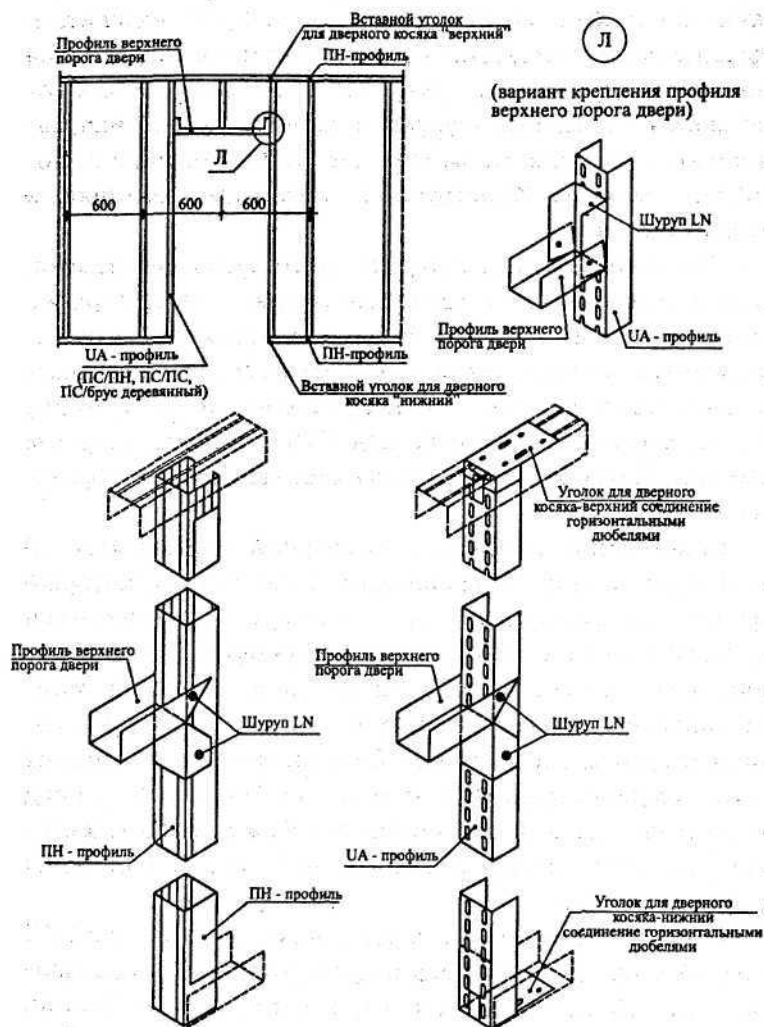
Рис. 1. Конструкция и узлы дверного проема
