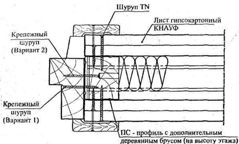
Рис. 2. Узел дверной коробки
