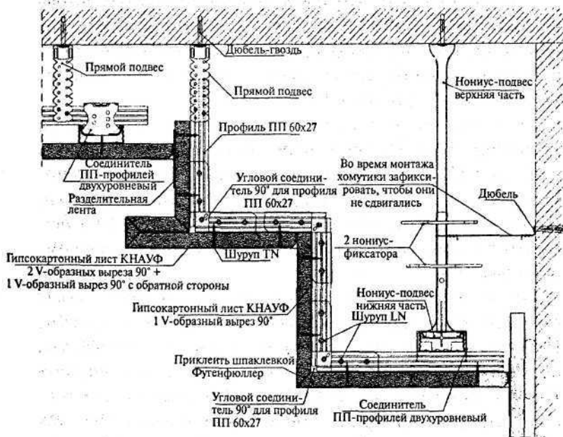
Рис. 10. Ступенчатый карниз
