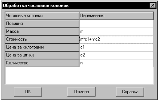
Рис. 10.4. Диалог обработки числовых колонок
