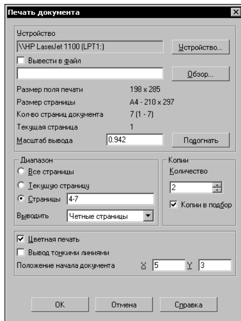
Рис. 10.12. Диалог настройки параметров печати
