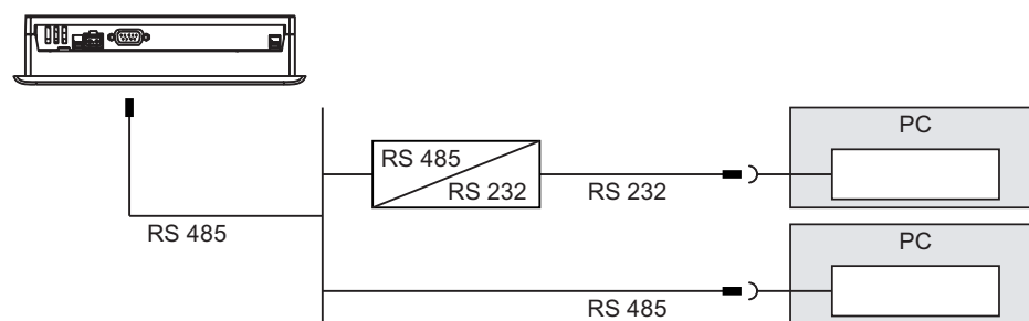
Рисунок 4-12 Подключение TP 177A к компьютеру проектирования
