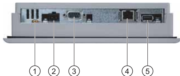
Рисунок 4-4 Интерфейсы устройства TP 177B PN/DP HMI
