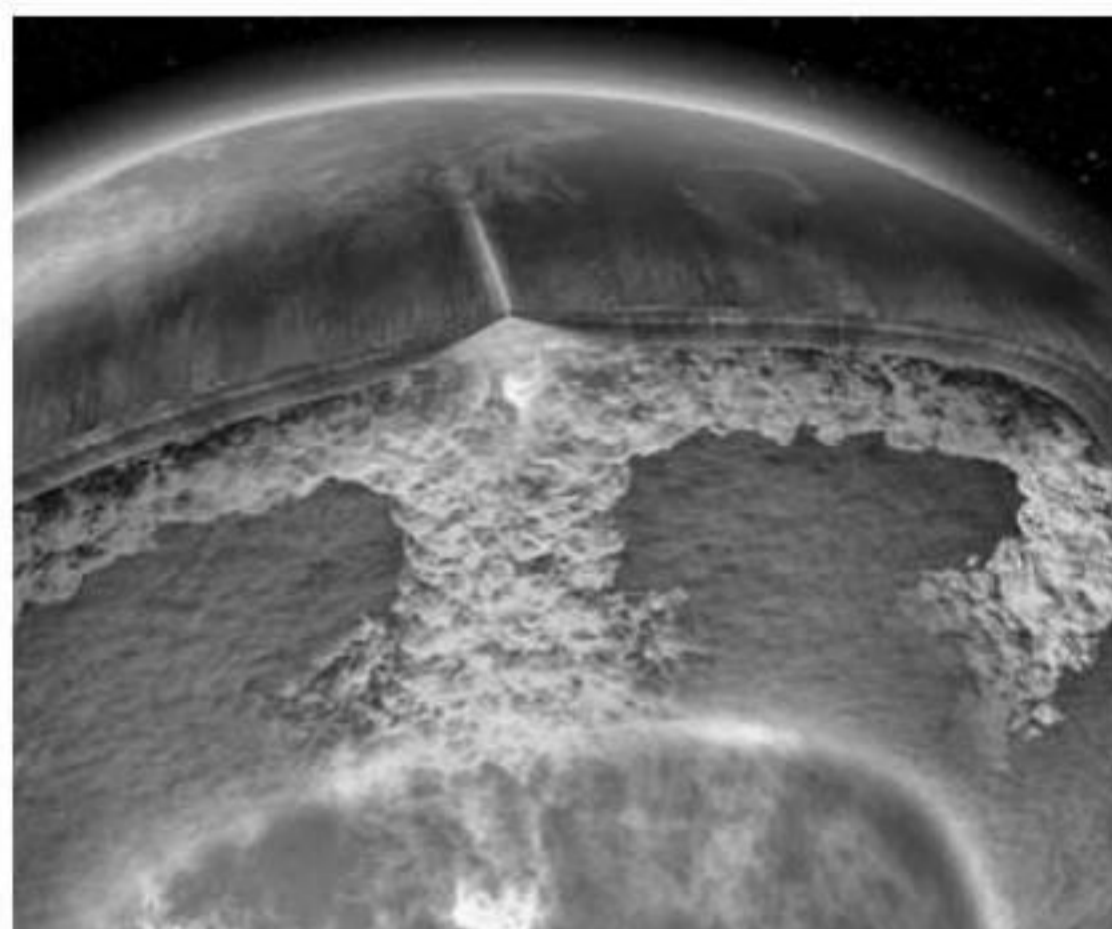
Мантия Земли
