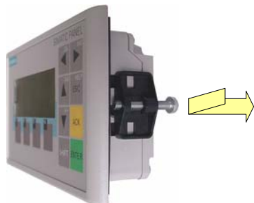
Рисунок 4-1 Установка зажимов в корпус OP 73micro.
