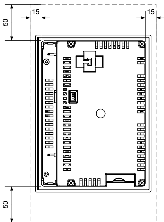
Рисунок 3-8 Зазоры при установке устройства НМІ
