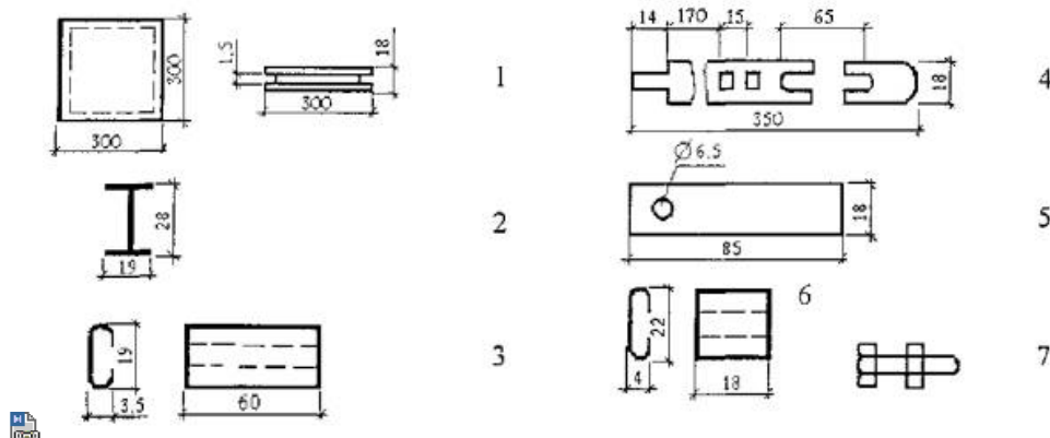
Рисунок 2 - Схемы крепления алюминиевых направляющих при устройстве подвесных потолков
