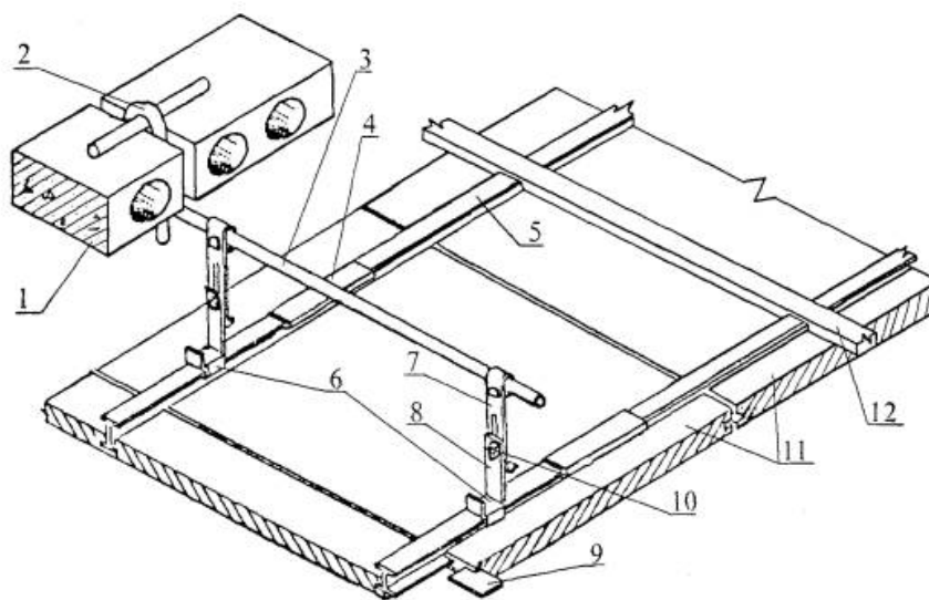
Рисунок 1 - Конструктивная схема подвесного потолка с лицевыми элементами из плит «Акмигран»
