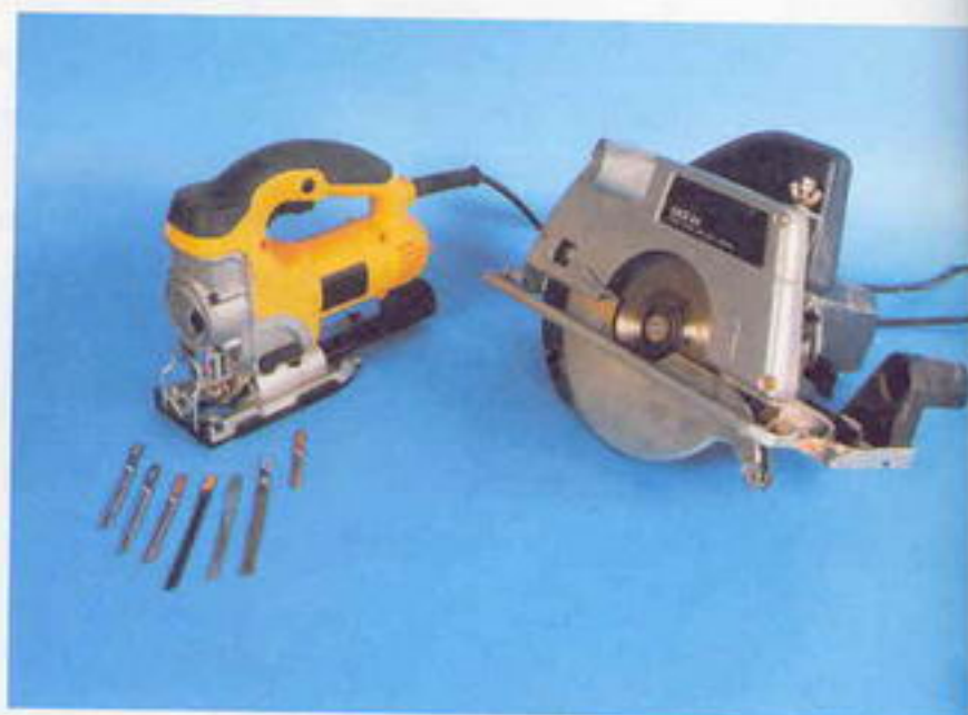
Электролобзик и циркулярная пила
