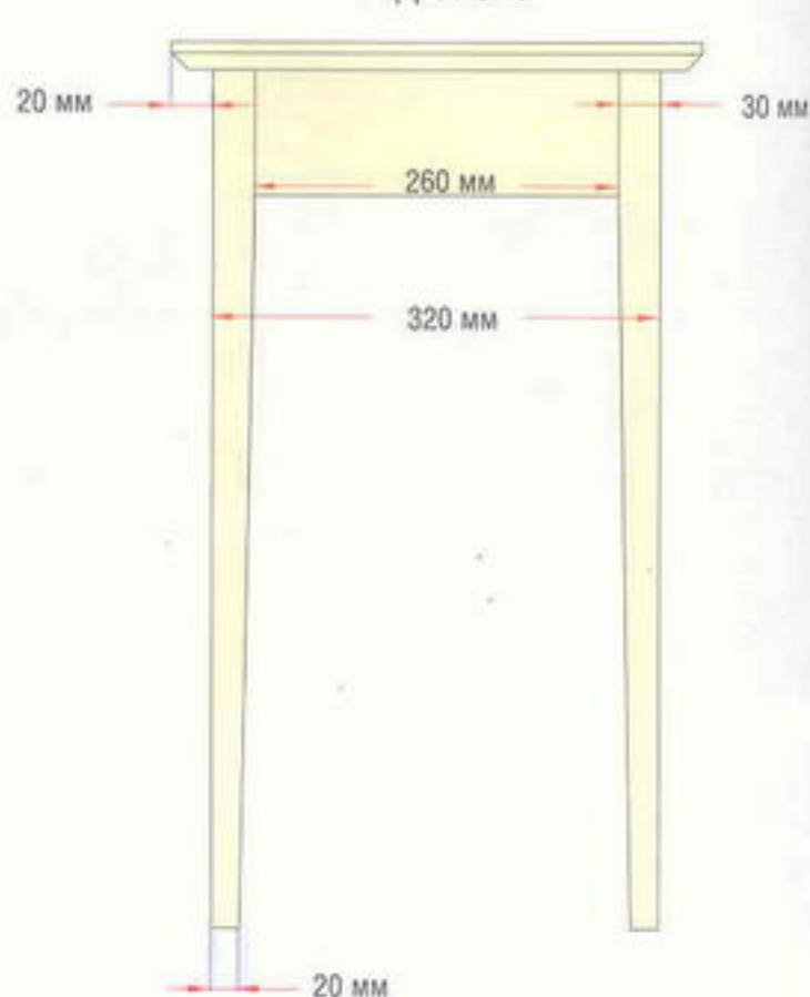
ВИД СБОКУ
