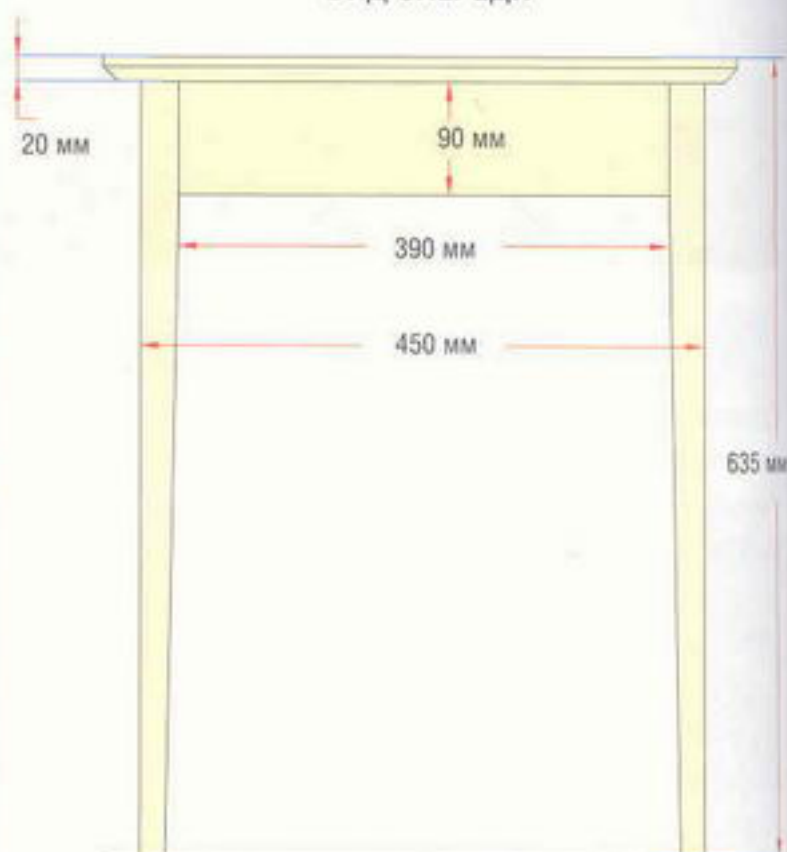
ВИД СПЕРЕДИ
