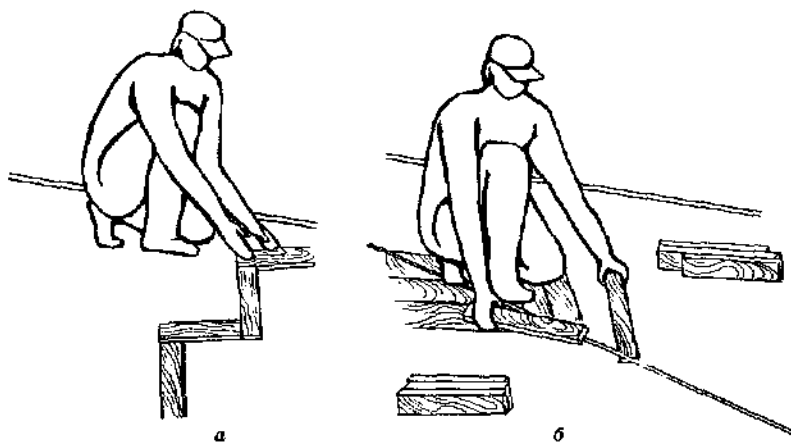
Рис. 75. Предварительная раскладка планок насухо: а — раскладка змейкой; б — укладка маячной елки
