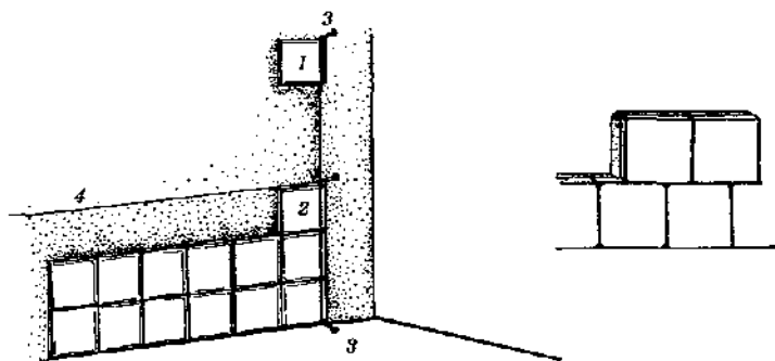
Рис. 66. Разметка основания стен и устройство маячных рядов: 1, 2 — первые маячные плитки; 3 — штыри; 4 — шнуры
