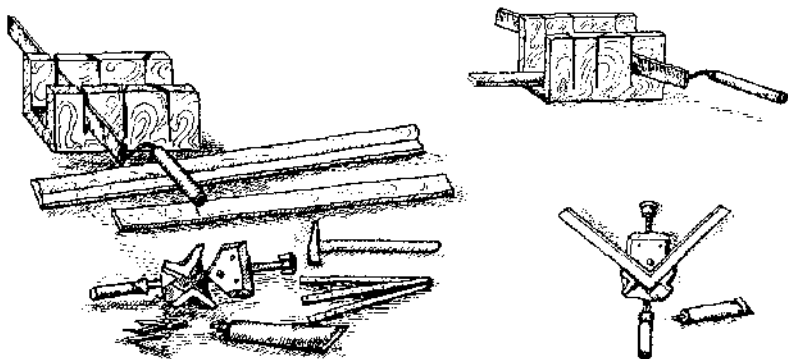
Рис. 31. Порядок изготовления багета
