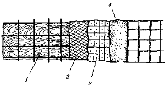
Рис. 60. Подготовка деревянного основания пола под облицовку плитками: 1 — деревянный настил; 2 — арматура или металлическая сетка; 3 — гидроизоляционный слой (рубероид); 4 — цементная штукатурка или бетон
