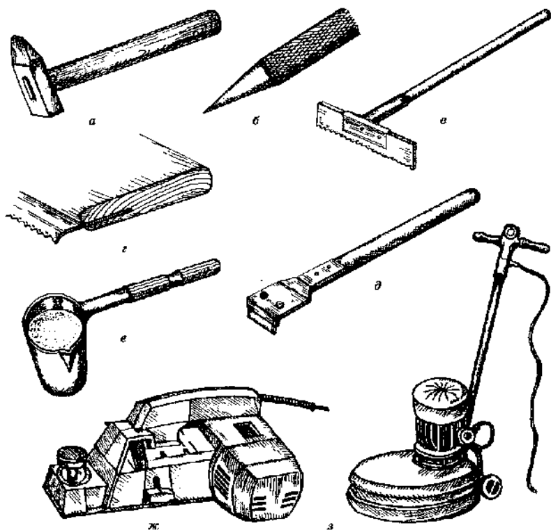
Рис. 71. Инструменты для паркетных работ: а — паркетный молоток; б — добойник; в — гребенка; г, д — цикли с короткой и длинной ручками; е — мерный черпак; ж — ручной электрический рубанок; з — полотерная машина
