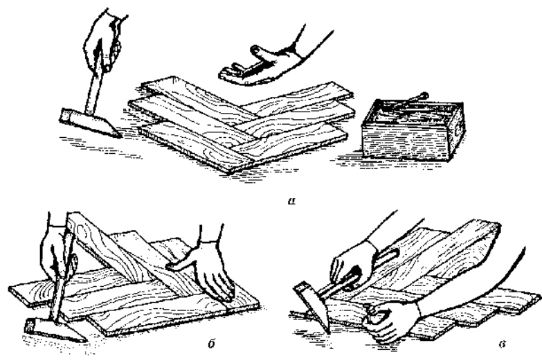
Рис. 80. Настилка штучного паркета «в елку» на гвоздях: а — посадка ударом молотка продольной кромки планки; б — посадка ударом молотка торцевой кромки планки; в — забивка гвоздя в паз планки
