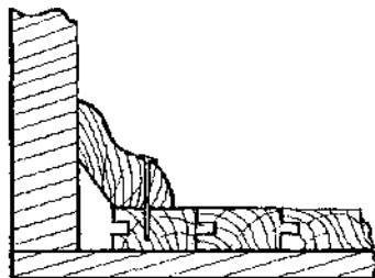
Рис. 85. Крепление галтели к паркету
