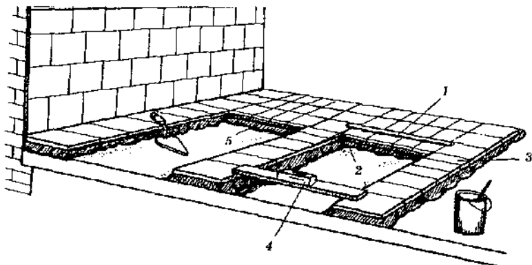
Рис. 63. Укладка плиток захватками: 1 — правило; 2 — раствор; 3 — маячный ряд; 4 — уровень; 5 — шнур
