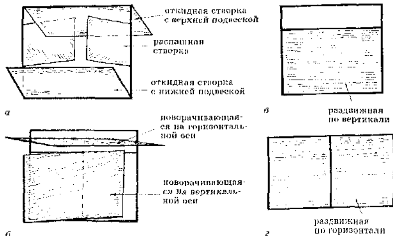
Рис. 8. Типы оконных переплетов: а — шарнирные створка (распашные или откидные, открывающиеся внутрь или наружу); б — створки, вращающиеся на подпятниках; в — подъемные створки; г — раздвижные створки.
