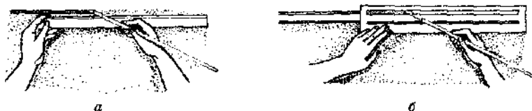
Рис. 49. Отводка филенки: а — по линейке с фаской; б — по трафарету
