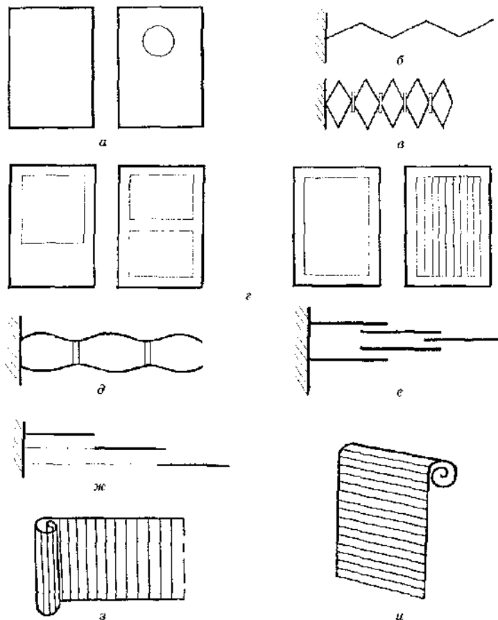
Рис. 7. Конструкции дверей: а — щитовые; б — складчатые; в — жесткая, гармошкой; г — филечатые; д — мягкая, гармошкой; е — телескопическая двусторонняя; ж — телескопическая односторонняя; з — складчатая вертикально; и — складчатая горизонтально
