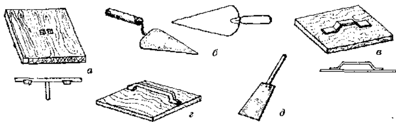
Рис. 40. Инструменты для штукатурных работ: а — сокол; б — штукатурная лопатка; в — полутерки; г — терка; д — скрепки
