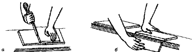
Рис. 61. Подготовка плиток: а — резка; б — раскалывание по разметке
