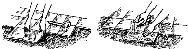
Рис. 58. Укладка и припрессовка поливинилхлоридных плиток
