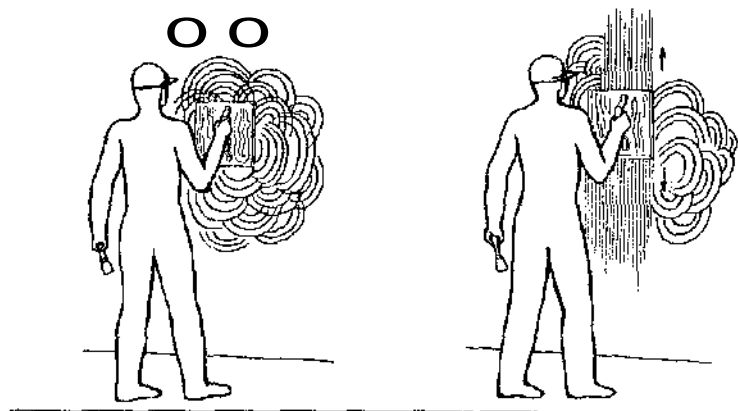
Рис. 43. Затирка штукатурки теркой на стене: а — вкруговую; б — вразгонку
