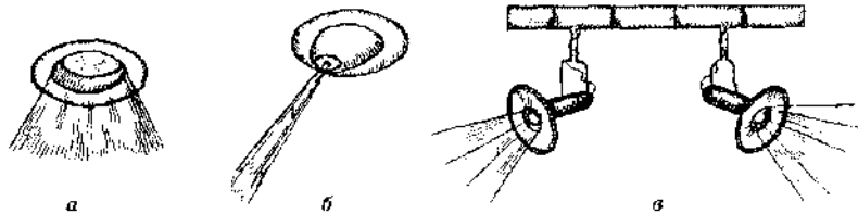
Рис. 35. Точечные светильники: а — утопленный точечный; б — поворотный; в — на шинном проводе
