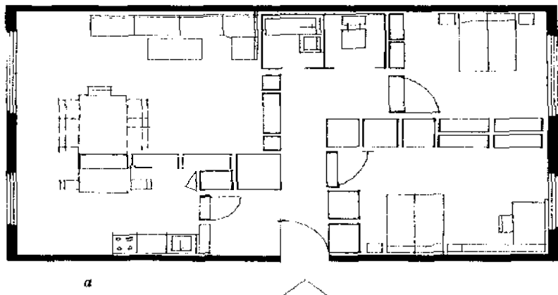
Рис. 1. Масштабный план квартиры: а — исходный план
