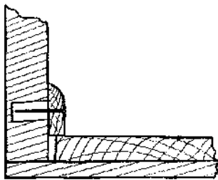
Рис. 84. Крепление плинтуса к стенам
