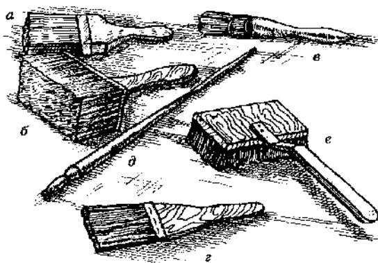
Рис. 45. Кисти для малярных работ: а — побелочная; б — макловица; в — ручник; г — флейца; д — филеочная; е — торцовка •
