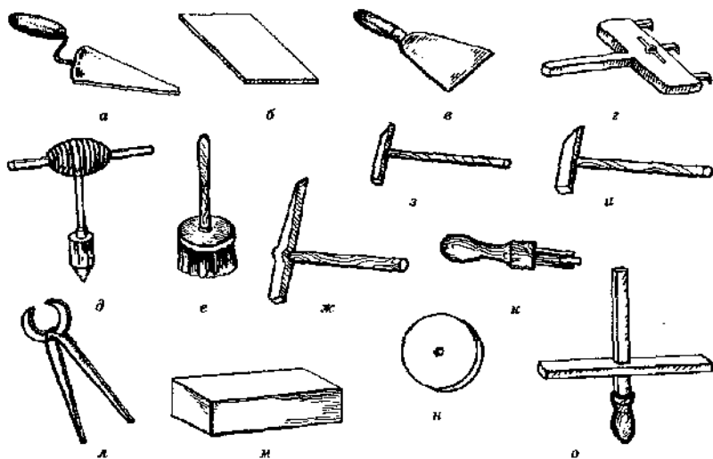
Рис. 59. Инструменты для плиточных работ: а — штукатурная лопатка; б — стальной шпатель; в — резиновый шпатель; г — царька; д — отвес массой 150 г; е — кисть; ж — молоток массой 600 г; з, и — плиточные молотки массой 60 г и 80 г; к — стальной резец с наконечником из твердого сплава; л — клещи; м — карборундовый брусок; н — карборундовый круг; о — шаблон
