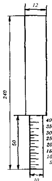
Рис. 72. Деревянный пестик для определения густоты мастики
