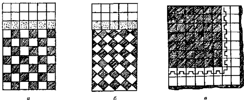
Рис. 64, Рисунок настилки пола: а — прямой; б — диагональный; в — с фризом
