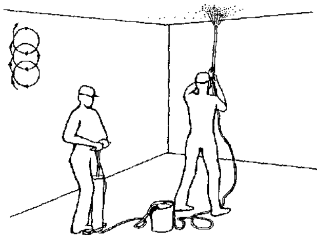
Рис. 50. Схема движения форсунки краскопульта или пульверизатора пылесоса
