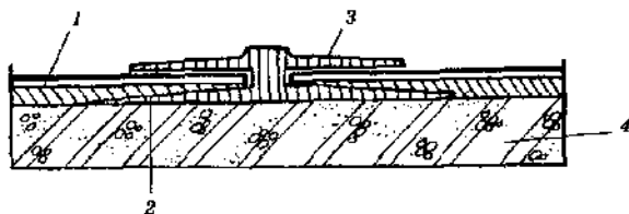
Рис. 56. Соединение линолеума на теплозвукоизолирующей подоснове с порошком в дверном проеме: 1 — линолеум; 2 — клей или мастика; 3 — порожек; 4 — бетонное основание
