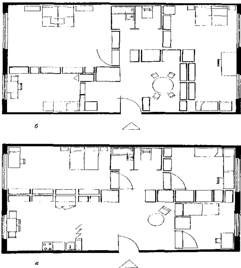
Рис. 1. Масштабный план квартиры (продолжение): б, в — предполагаемые варианты перепланировки
