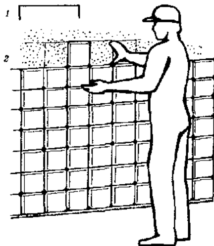
Рис. 67. Облицовка стен со швами: 1 — скоба; 2 — проверка ширины вертикальных и горизонтальных швов
