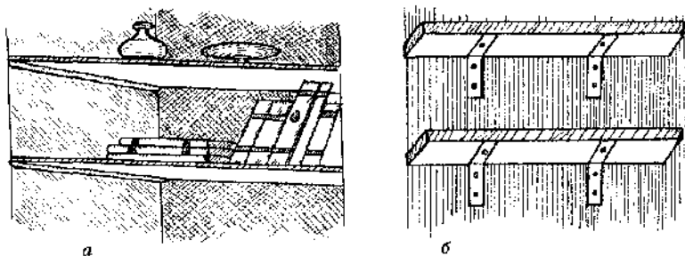
Рис. 23. Крепление полок: а — при помощи реек; б — при помощи металлических уголков
