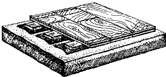
Рис. 73. Устройство основания под полы из паркетных досок
