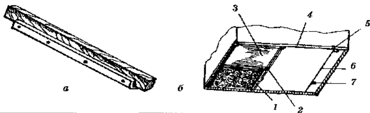
Рис. 55. Устройство песчано-цементной стяжки: а — установка маяков; б — установка направляющих реек: 1 — деревянная рейка; 2 — маяк; 3 — заглаженная заподлицо поверхность; 4 — уровень пола; 5 — штырь для шнура; 6 — шнур; 7 — маяки
