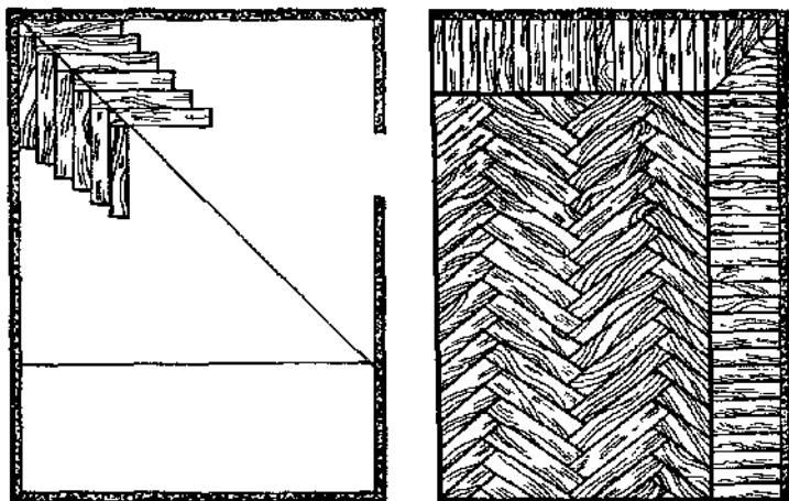
Рис. 77. Настилка паркета «в елку» с фризом
