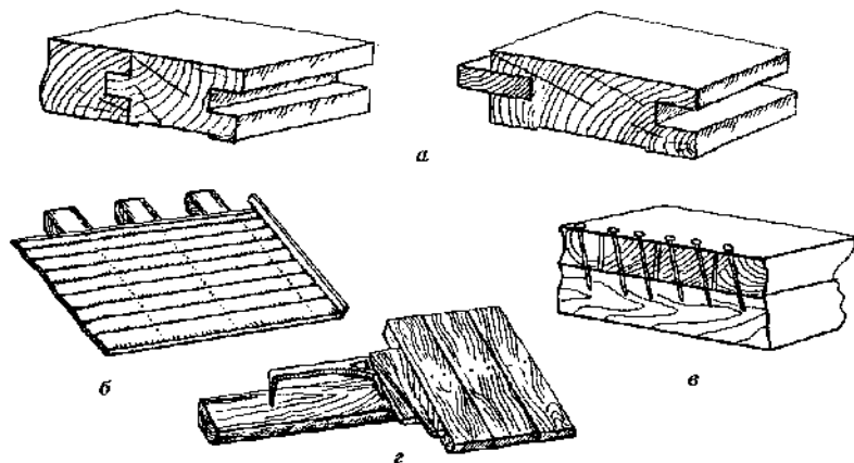
Рис. 68. Настилка дощатых полов: а — шпунтованные доски; б — стыкование досок; в — крепление досок гвоздями; г — сжатие досок с помощью скобы Смолякова
