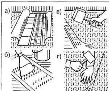
Рис. 15. Плоские металлические планки с шипами для соединения ковровых покрытий пола: а – стык; б – нанесение мастики; в, г – укладка
