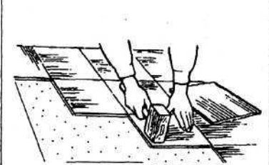
Рис. 13. Укладка и припрессовка поливинилхлоридных плиток
