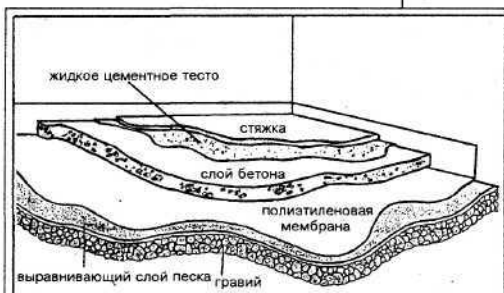
Рис. 2. Конструкция цементно-песчаной стяжки по бетонному основанию
