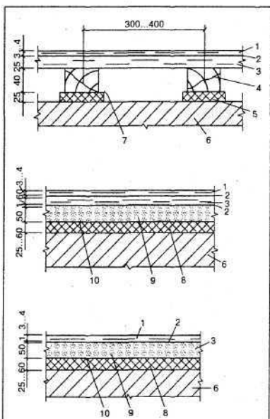
Рис. 20. Полы из сверхтвердых древесно-волокнистых плит: 1 - покрытие; 2 - клеевой слой; 3 - основание пола из досок или древесностружечных плит; 4 - лаги 40×80 мм; 5 - звукоизоляционные ленточные прокладки из древесно-волокнистых плит; 6 - несущая плита перекрытия; 7 - слой толя; 8 - звукоизоляционный сплошной слой; 9 - стяжка из легкого бетона; 10 - слой толя или пергамина
