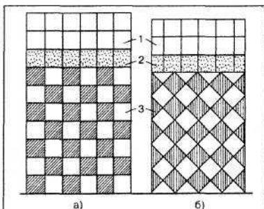
Рис. 9. Двухцветный пол из керамических плиток:
