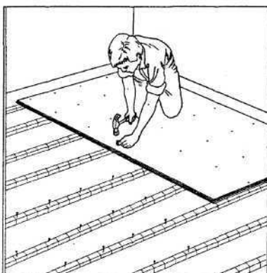
Рис. 21. Устройство пола из древесно-волокнистых плит
