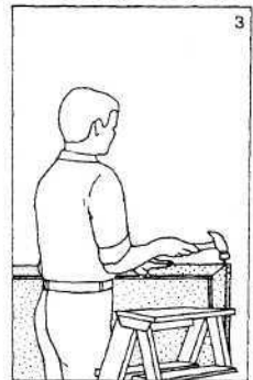
Рис. 25. Крепление дверной коробки к стене
