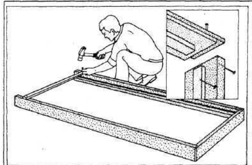
Рис. 24. Сборка и установка дверной коробки
