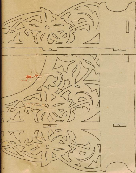
Рис. 29. Настольная рамочка для зеркала.
