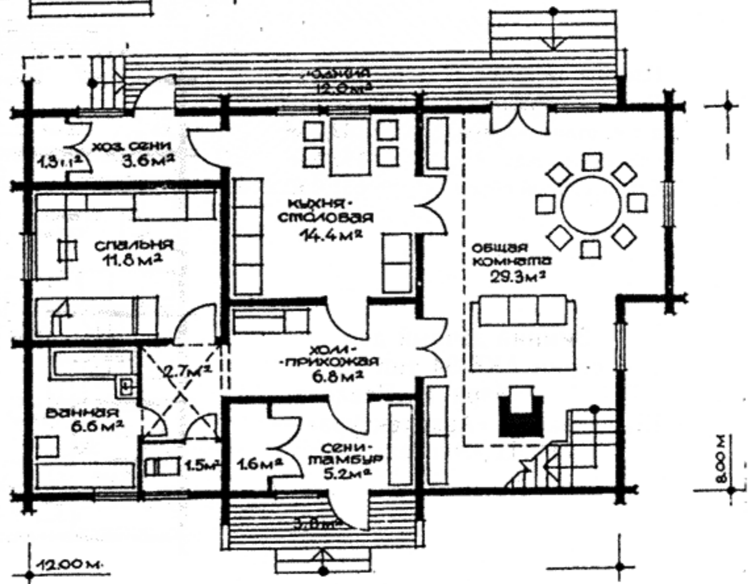
План I этажа
