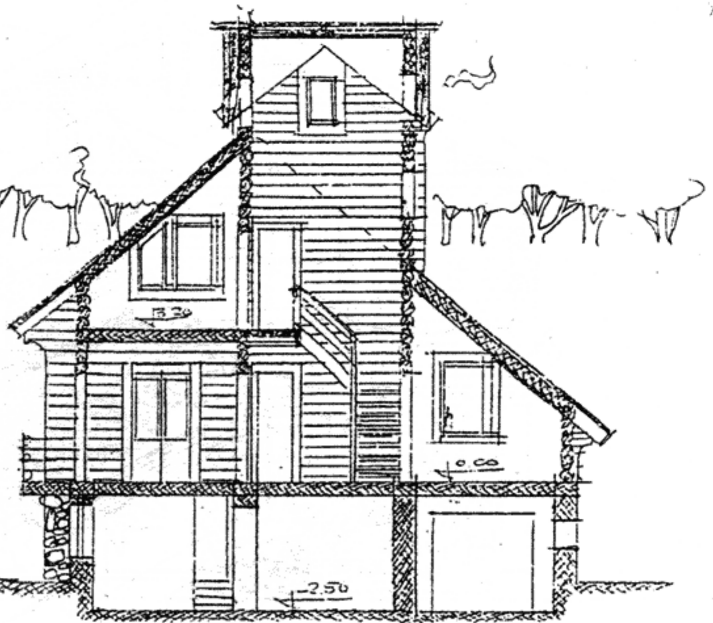
Разрез
