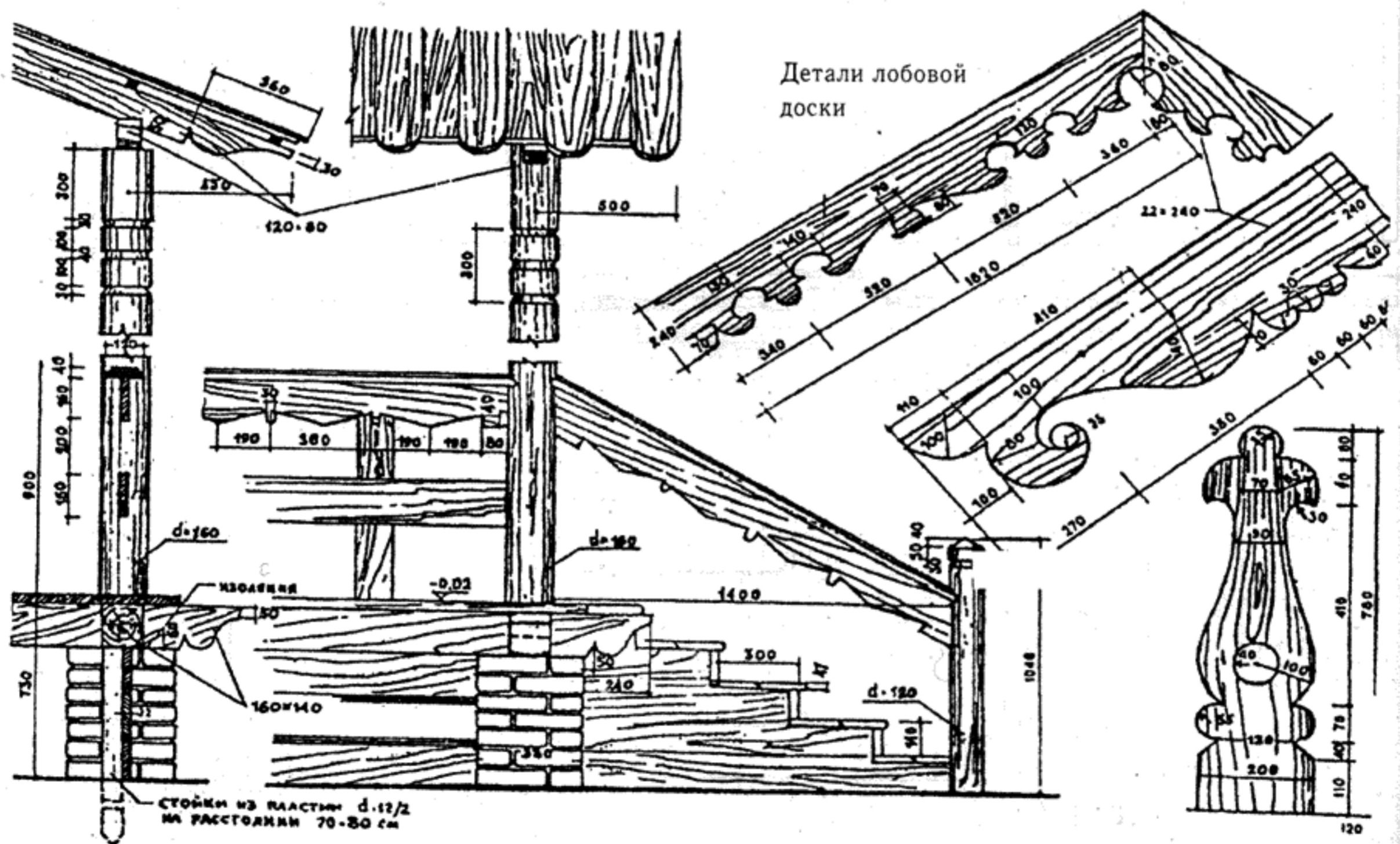
Детали крыльца
