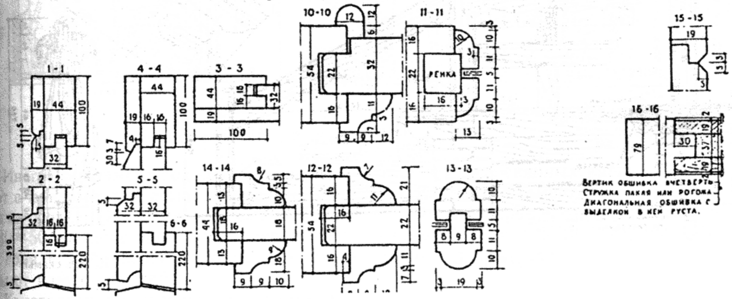
Двери для жилища и надворных построек. Проектная разработка школы-мастерской акад. И. Жолтовского, 1949 г.
