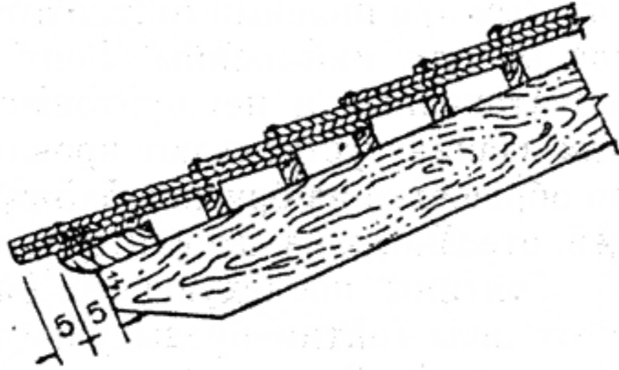
Устройство свеса
