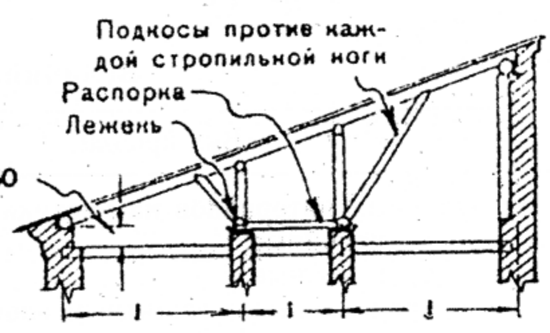
Схемы стропил односкатных кровель:
