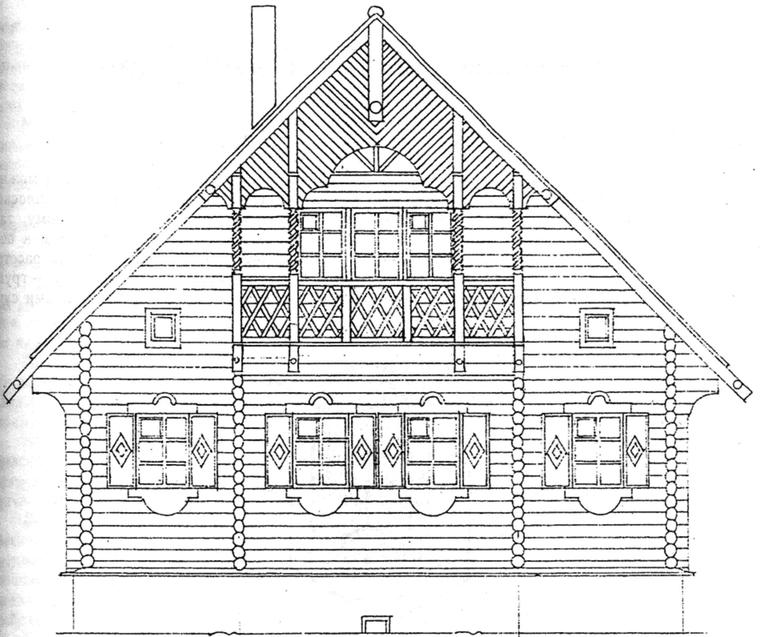
Резные детали деревянного дома-экспоната на Строительной выставке Росстройэкспо в Москве. Арх. М. Гурари, констр. Ф. Межуева. КБ редакции «Архитектура». Строительство — «Эколес» (Кострома), «Русский мастер» (Москва)
