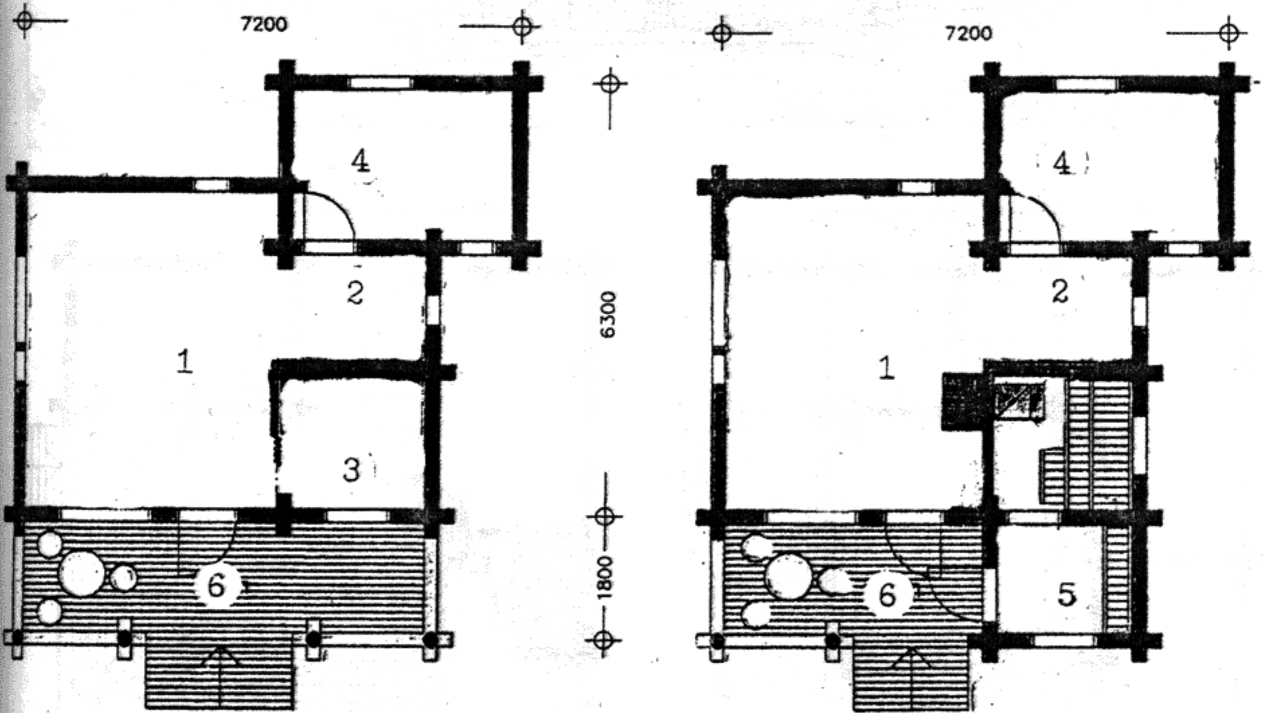
План I этажа (вариант)
