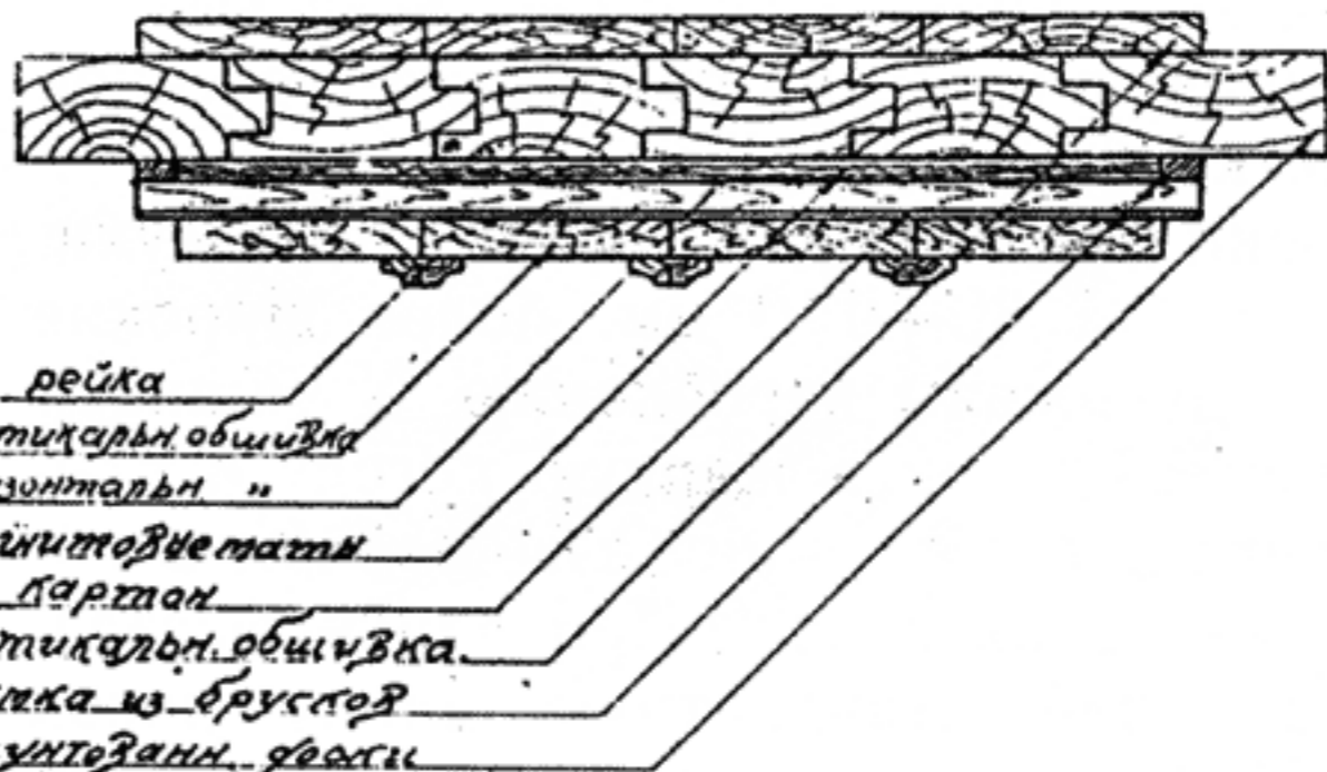
Вариант конструкции сборных щитов
