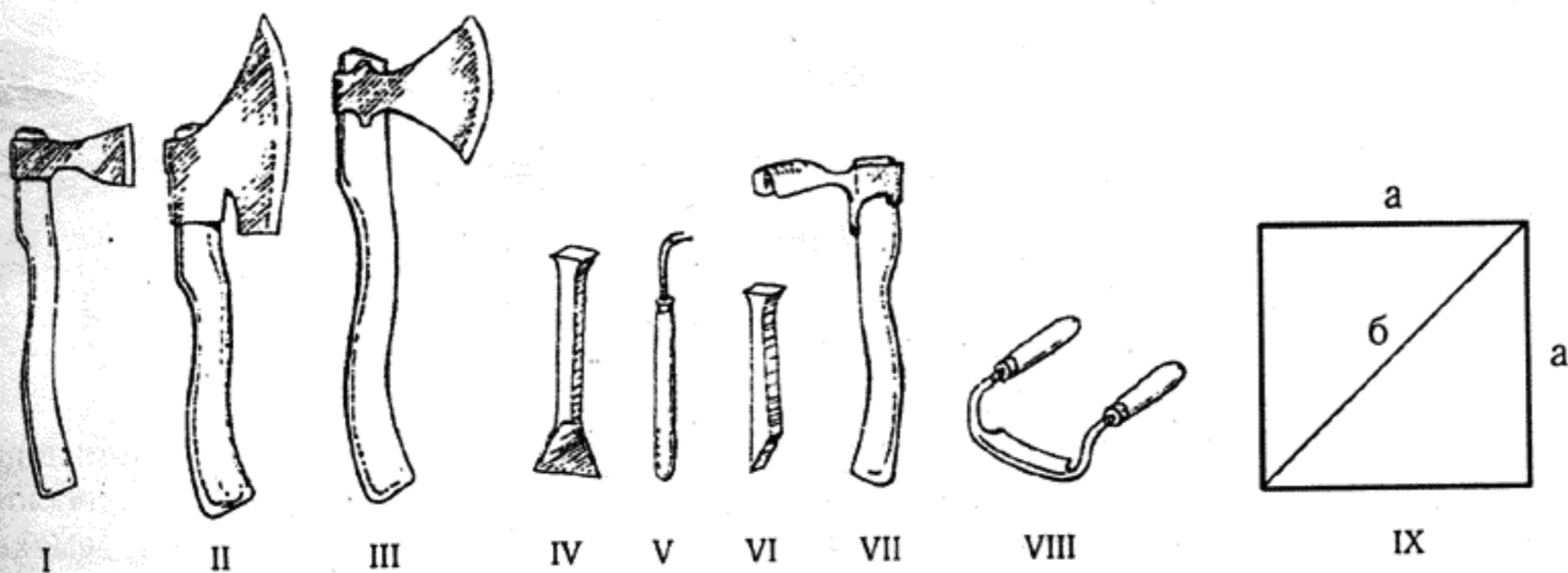
Инструмент плотника:
