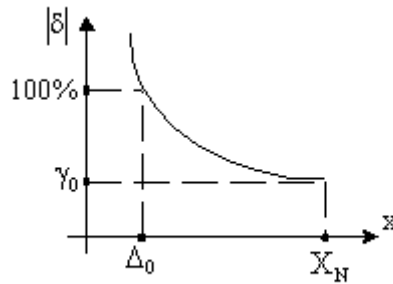
Рисунок 8.1 – Рабочий диапазон средства измерения
