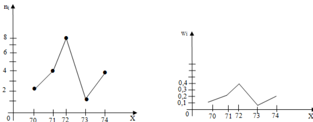
Рисунок 3.2 – Полигон частот и полигон относительных частот
