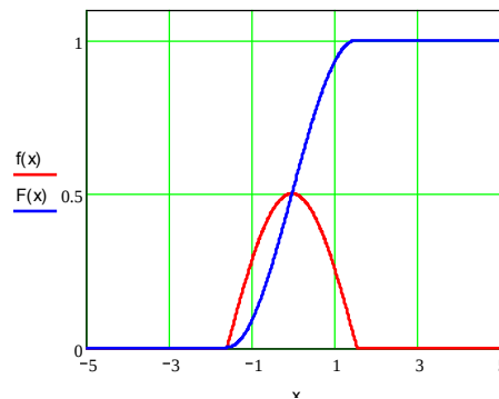
Рисунок 2.4 – График плотности распределения f(x) и функции распределения F(x)
