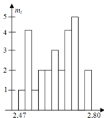
Рисунок 3.4 – Гистограмма частот
