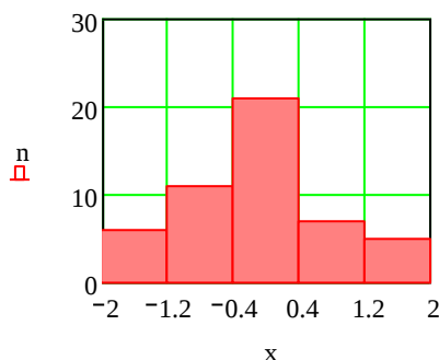
Рисунок 5.2 - Гистограмма
