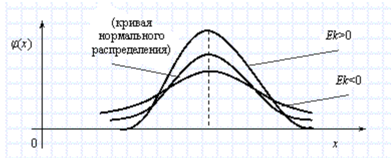
Рисунок 2.6 – Коэффициент эксцесса
