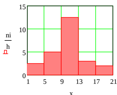
Рисунок 3.6 – Гистограмма
