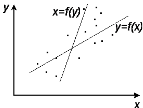
Рисунок 6.5 – Линейная регрессия
