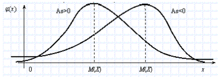
Рисунок 2.5 – Коэффициент асимметрии
