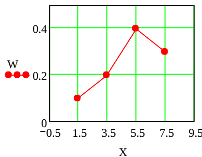
Рисунок 3.3 – Полигон относительных частот
