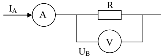
Рисунок 7.1 – Измерение мощности по методу амперметра и вольтметра (вариант 1)
