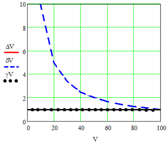
Рисунок 7.3 – Графики зависимостей абсолютной, относительной и приведённой погрешностей от результата измерений
