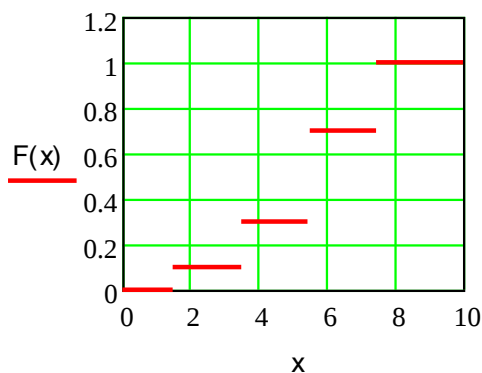
Рисунок 2.2 – Функция распределения
