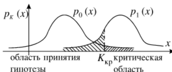
Рисунок 5.1 – Проверка статистической гипотезы
