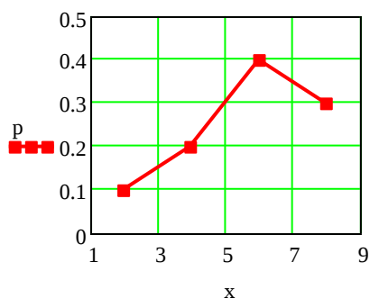
Рисунок 2.1 – Многоугольник распределения
