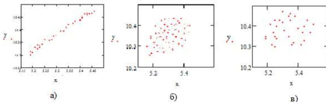
Рисунок 6.2 – Сила корреляции
