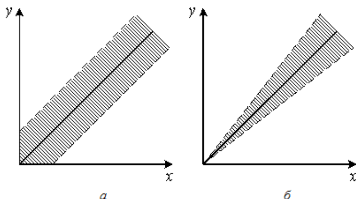
Рисунок 7.4– Аддитивная и мультипликативная погрешности
