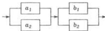
Рисунок 1.1 – Схема параллельного подсоединения блоков подсистем
