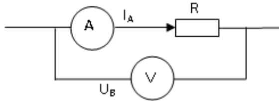
Рисунок 7.2 – Измерение мощности по методу амперметра и вольтметра (вариант 2)
